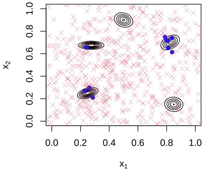
Population Monte Carlo
