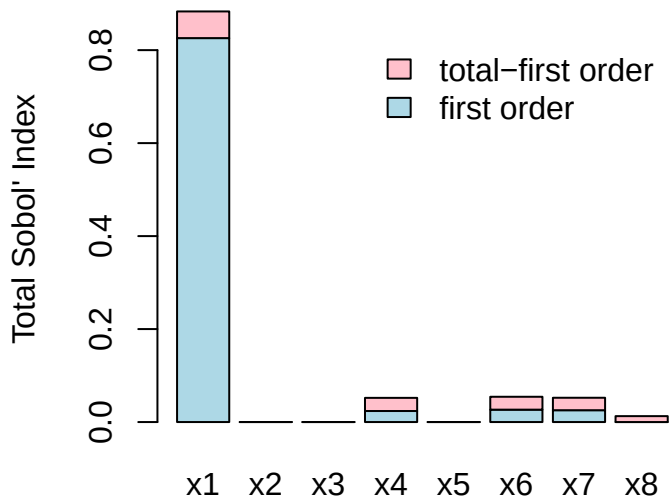
Sobol' Indices
