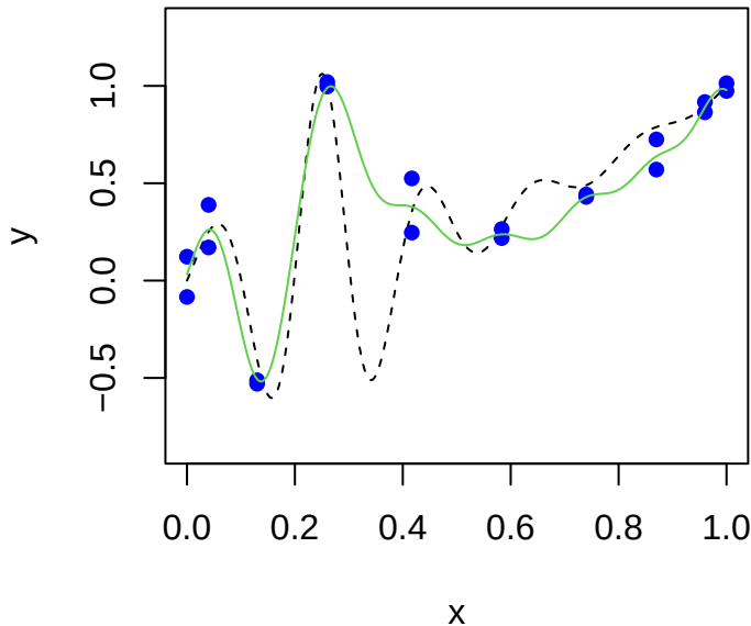
kernel ridge regression (D-optimal)
