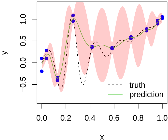
GP Regression (D-optimal)
