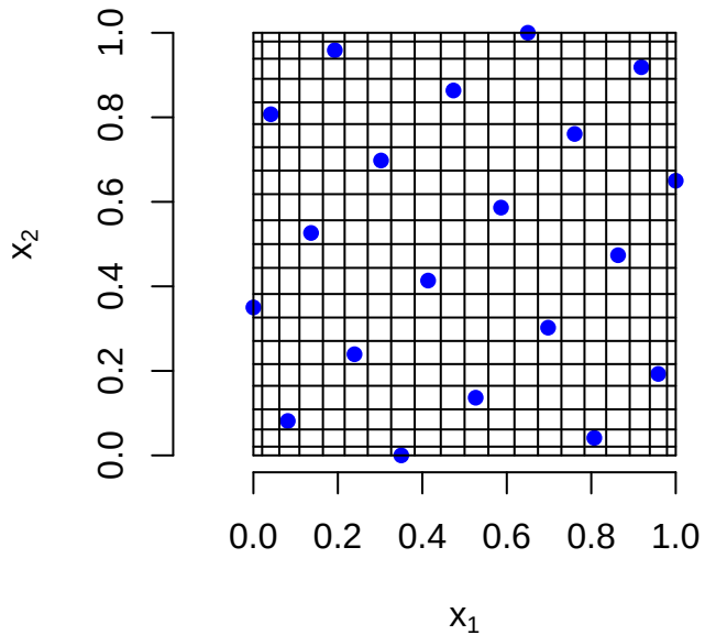
MaxPro(20,2)
