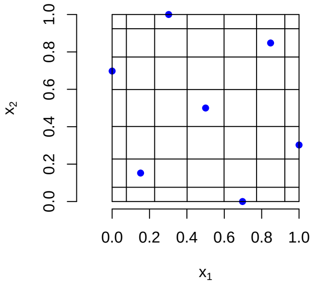
MaxPro(7,2)
