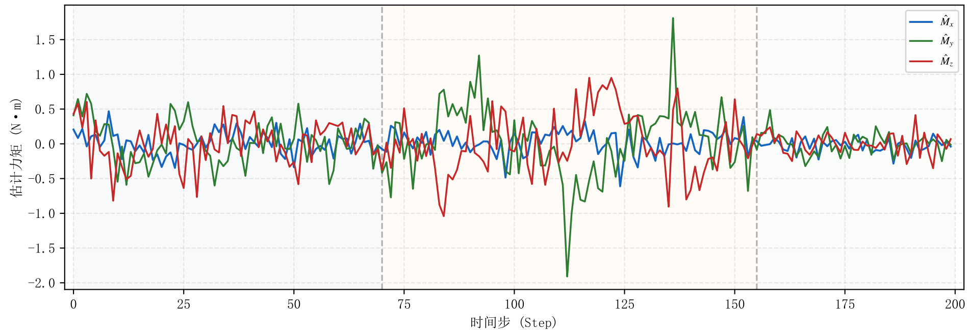
末端估计三轴力矩响应
