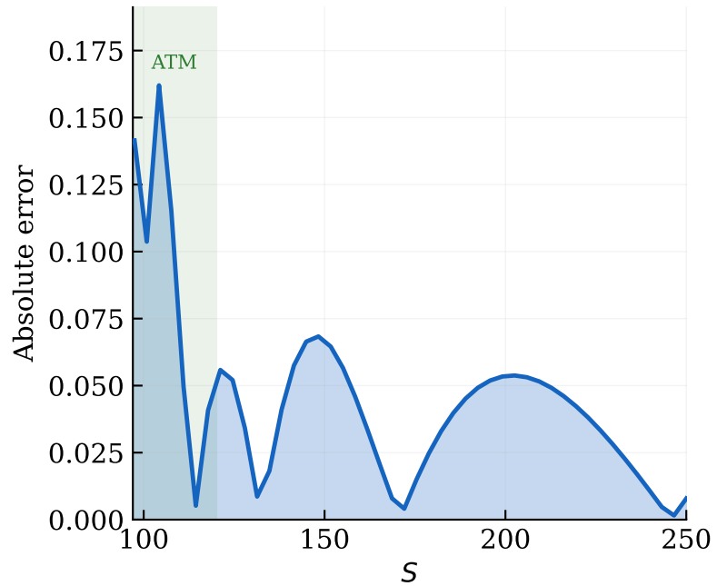
CEV ( \beta=0.5 )
