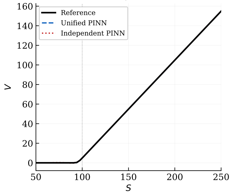
CEV ( \beta=0.5 )
