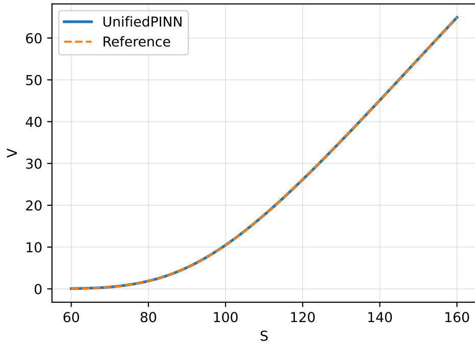
BSM
