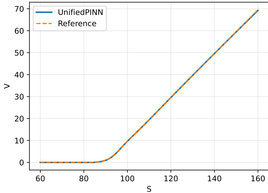
CEV (beta=0.5)
