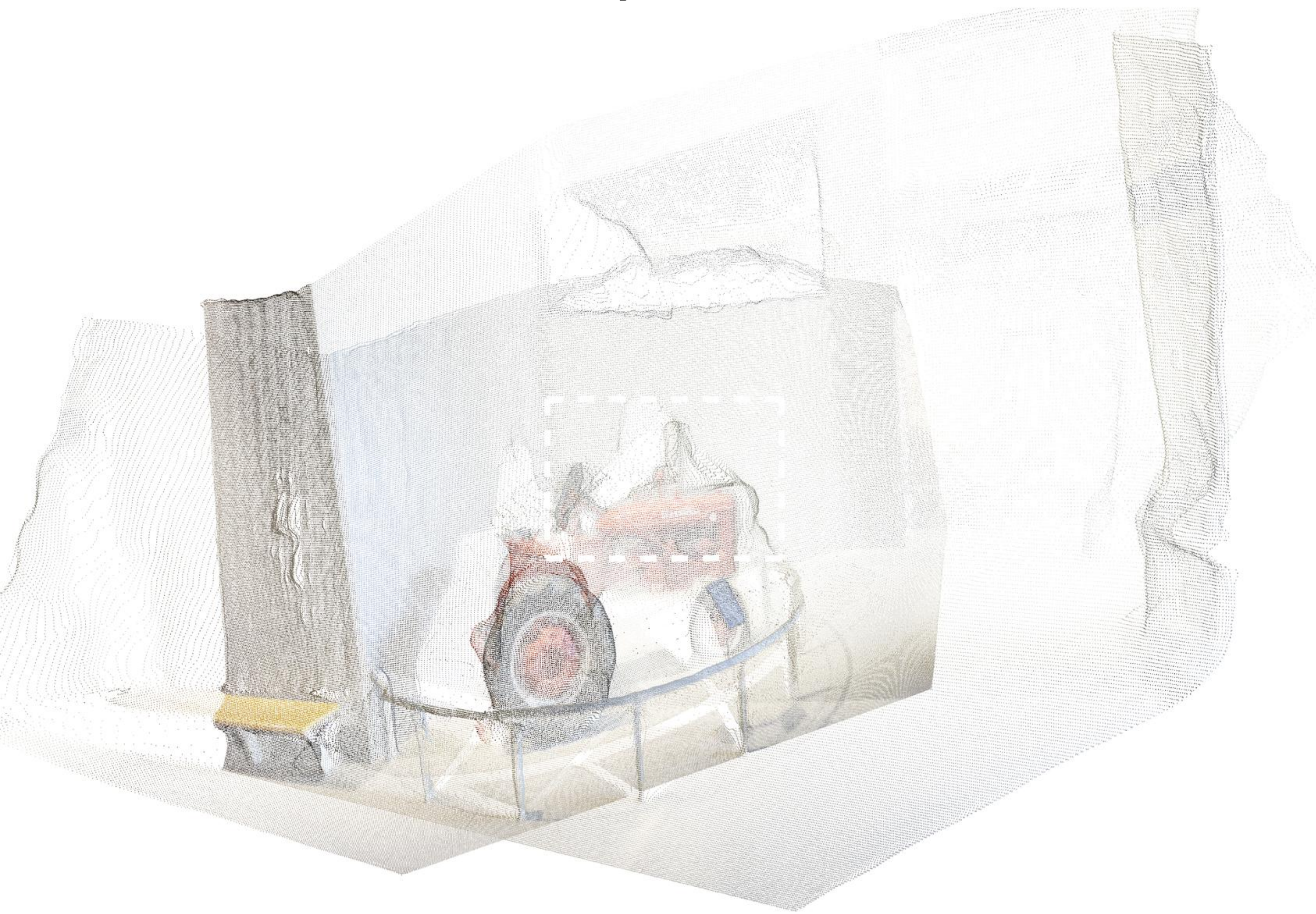
Sparse
