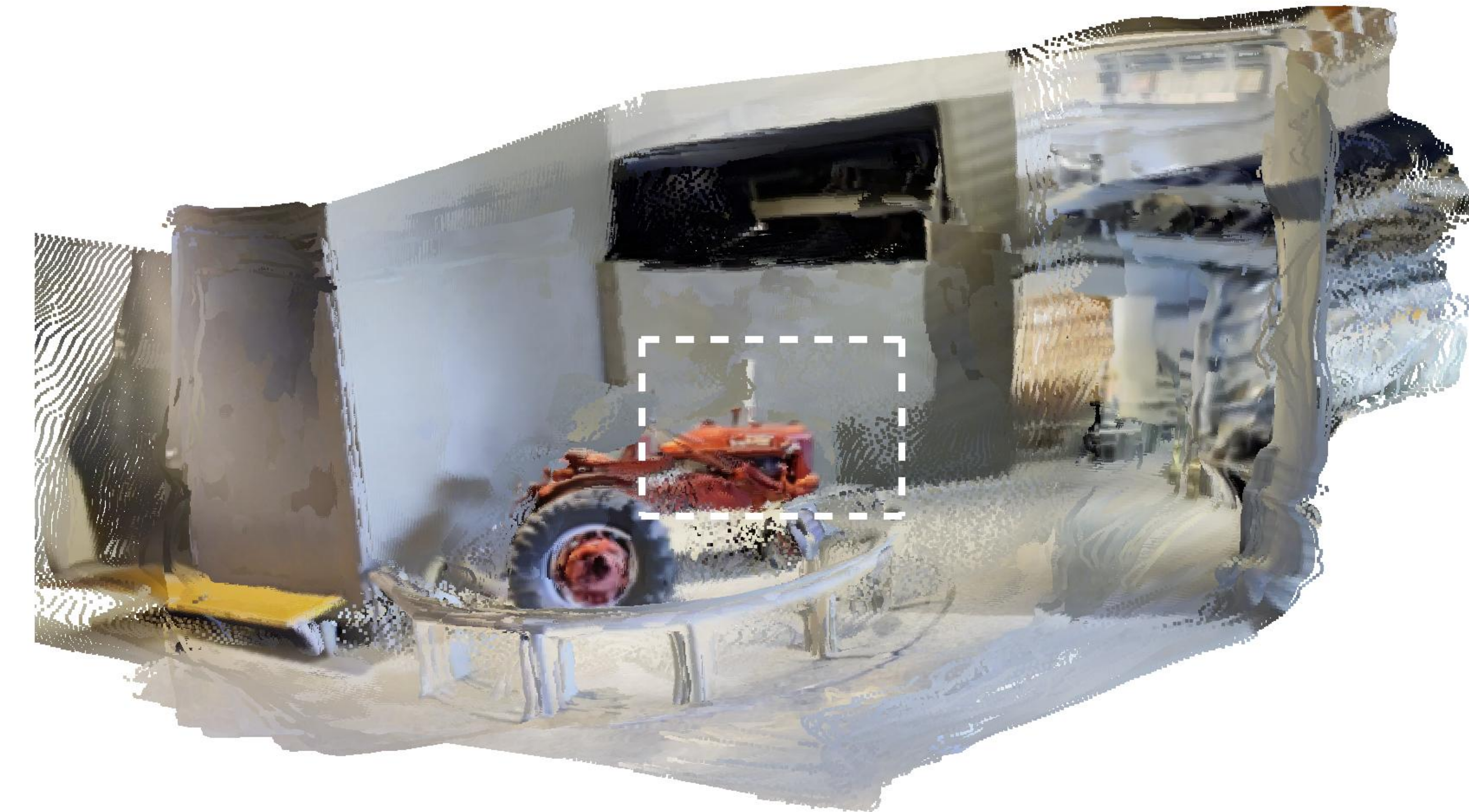
Ours
