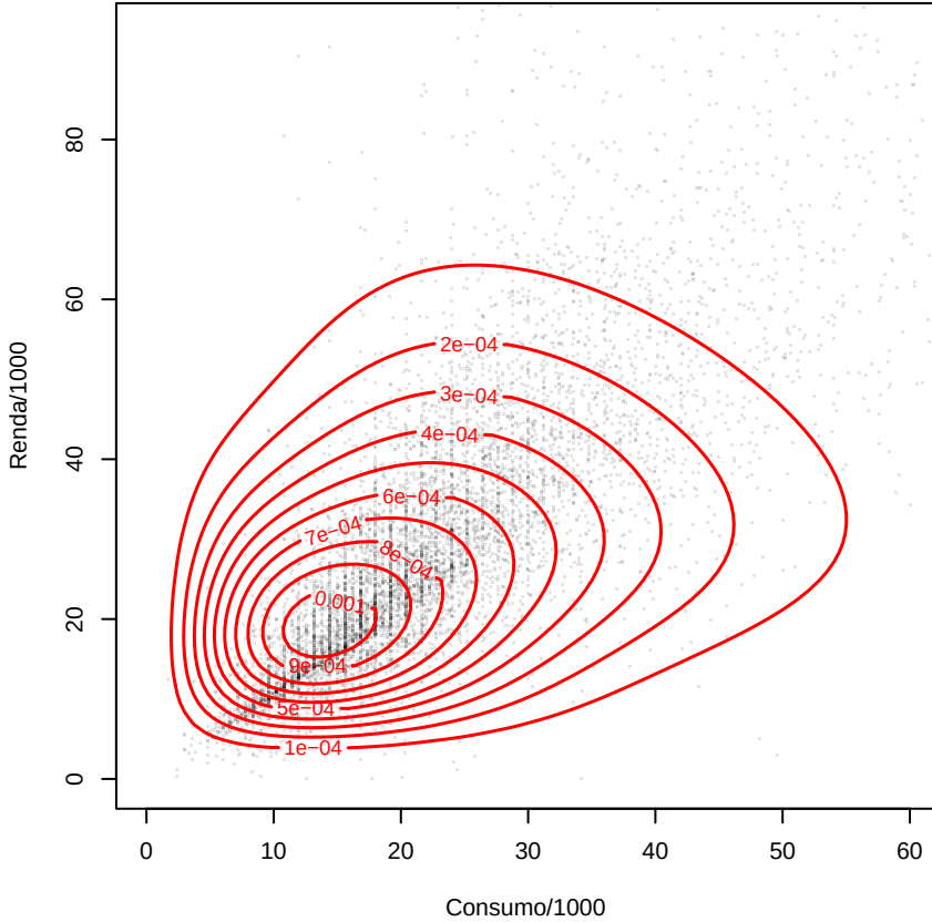
Dados e contornos do modelo ajustado
