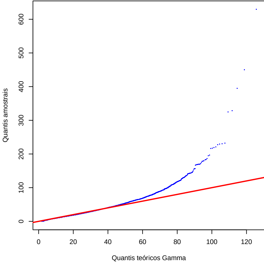
QQ-plot: Renda vs Gamma
