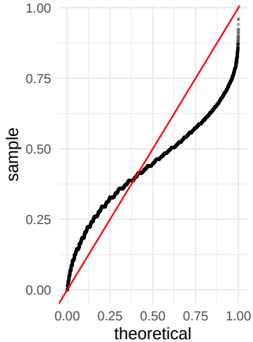
QQ Unif — Y
