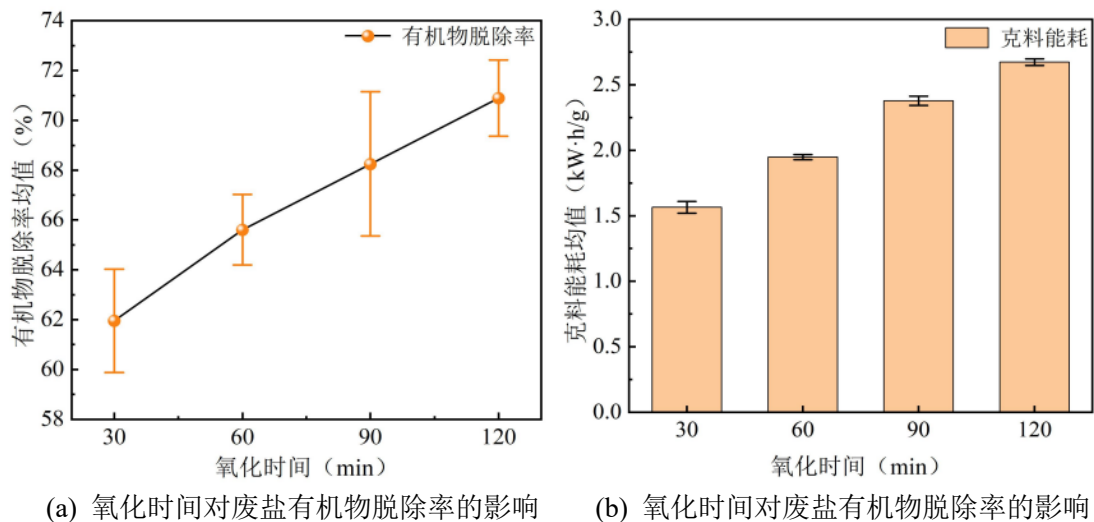
图 4.2 氧化时间对废盐有机物脱除效率及单位能耗的影响
