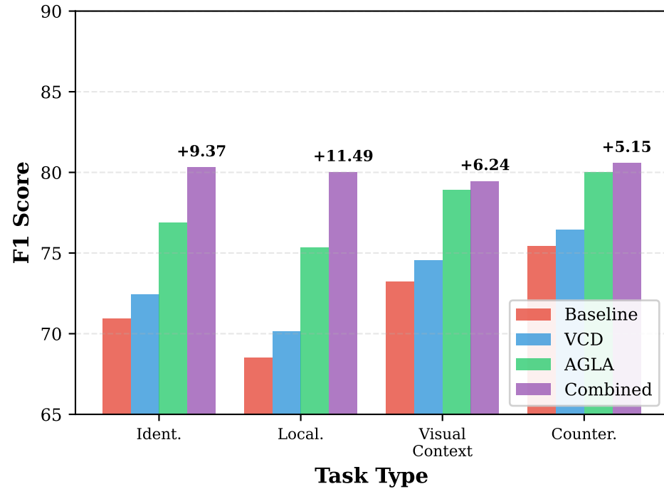
LLaVA-1.6
