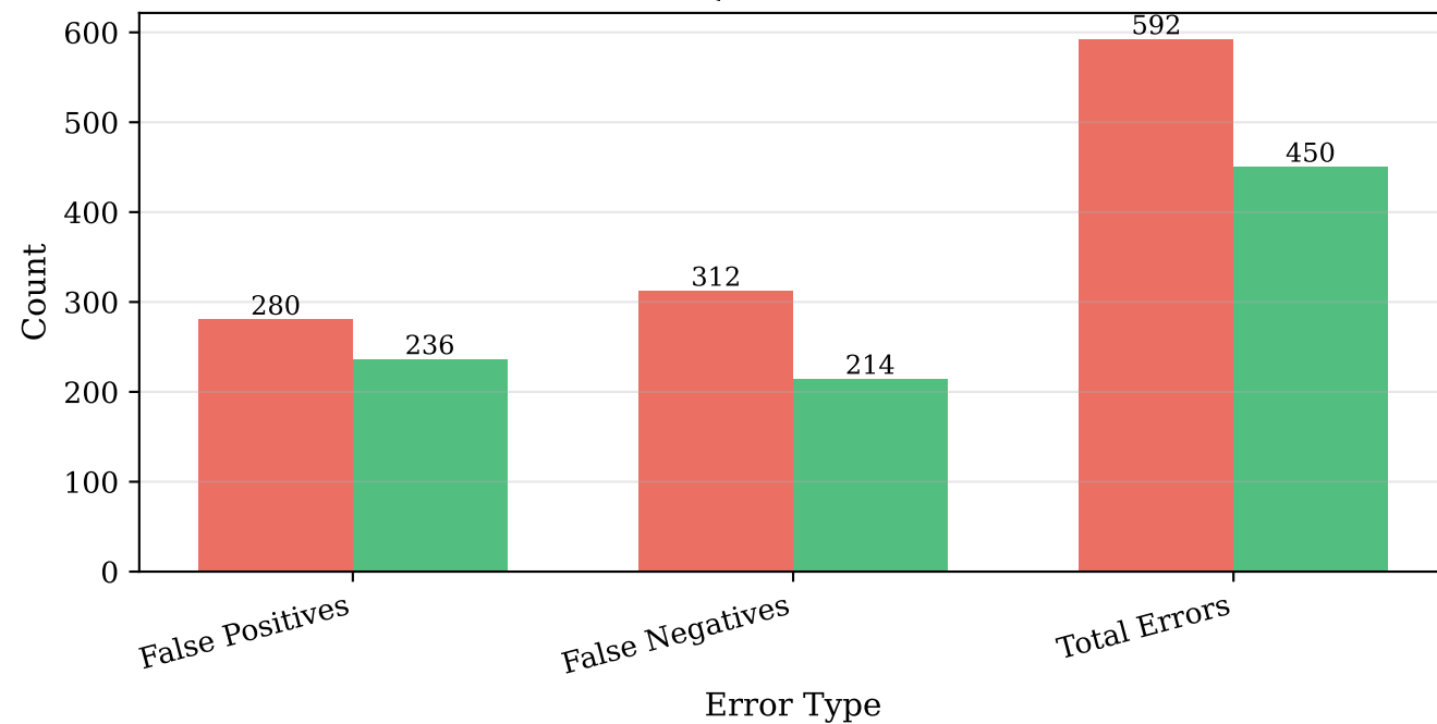
A-OKVQA: Error Counts
