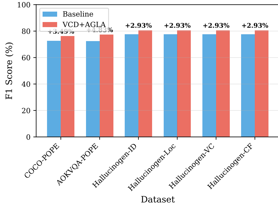
LLaVA-1.6-7B
