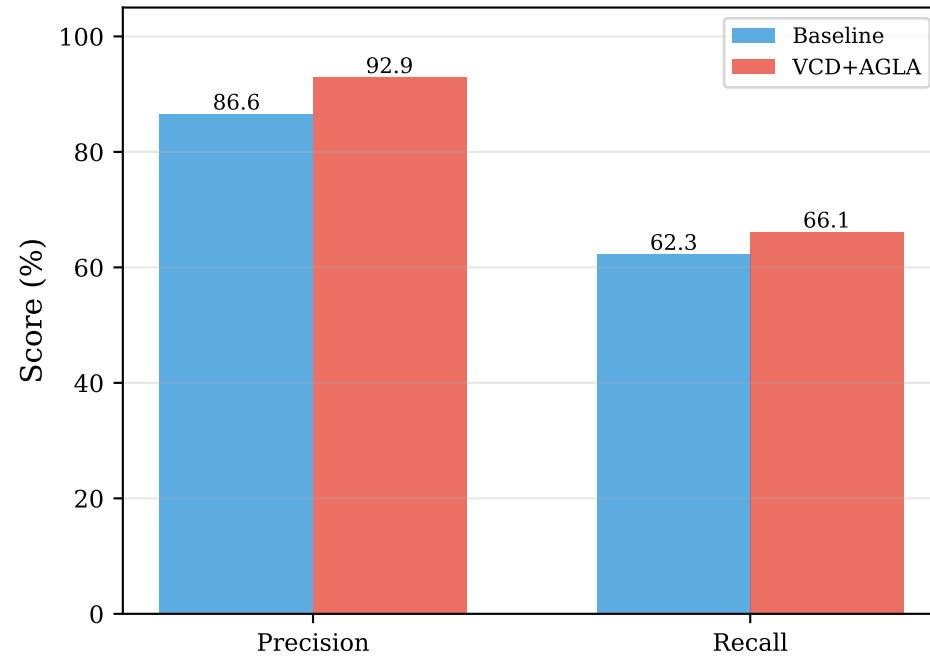
LLaVA-1.6-7B AOKVQA-POPE
