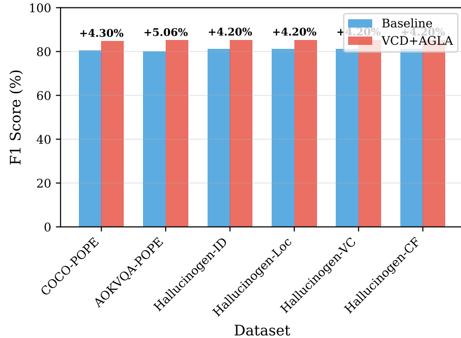
LLaVA-1.5-7B
