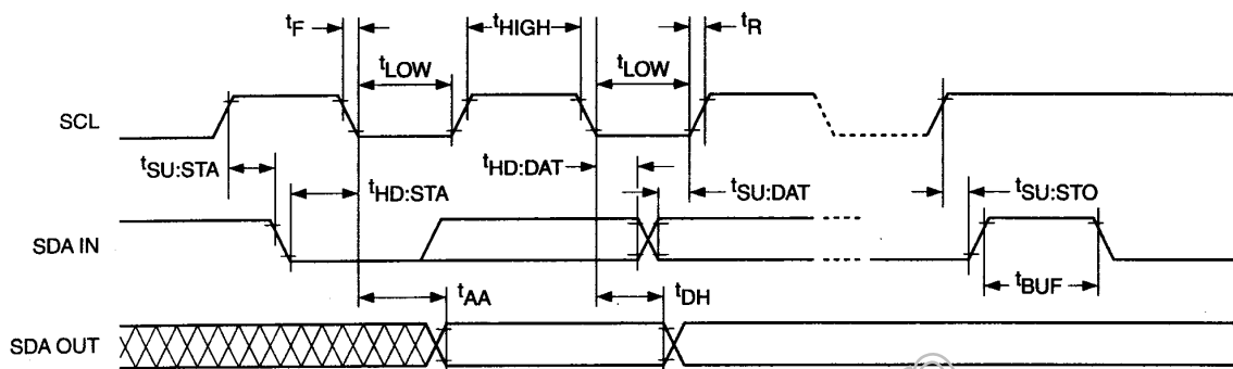
图 1 总线时序
