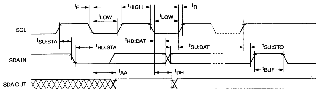
图 1 总线时序
