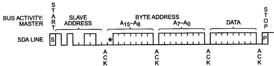
图 6 字节写时序
