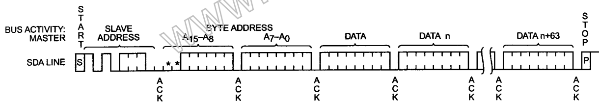
图 7 页写时序
