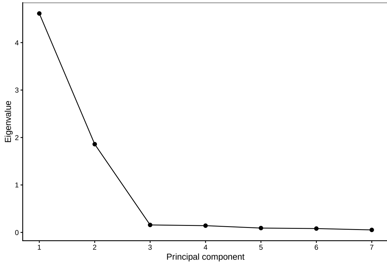
PCA eigenspectrum
