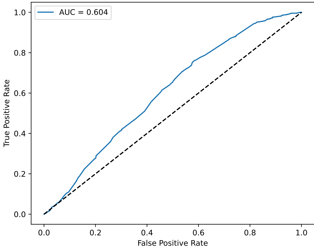
Krzywa ROC
