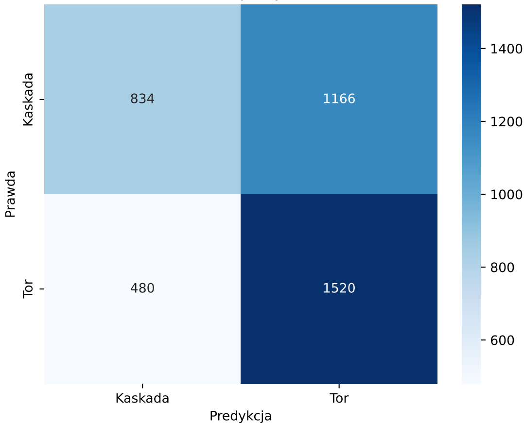
Macierz pomyłek
