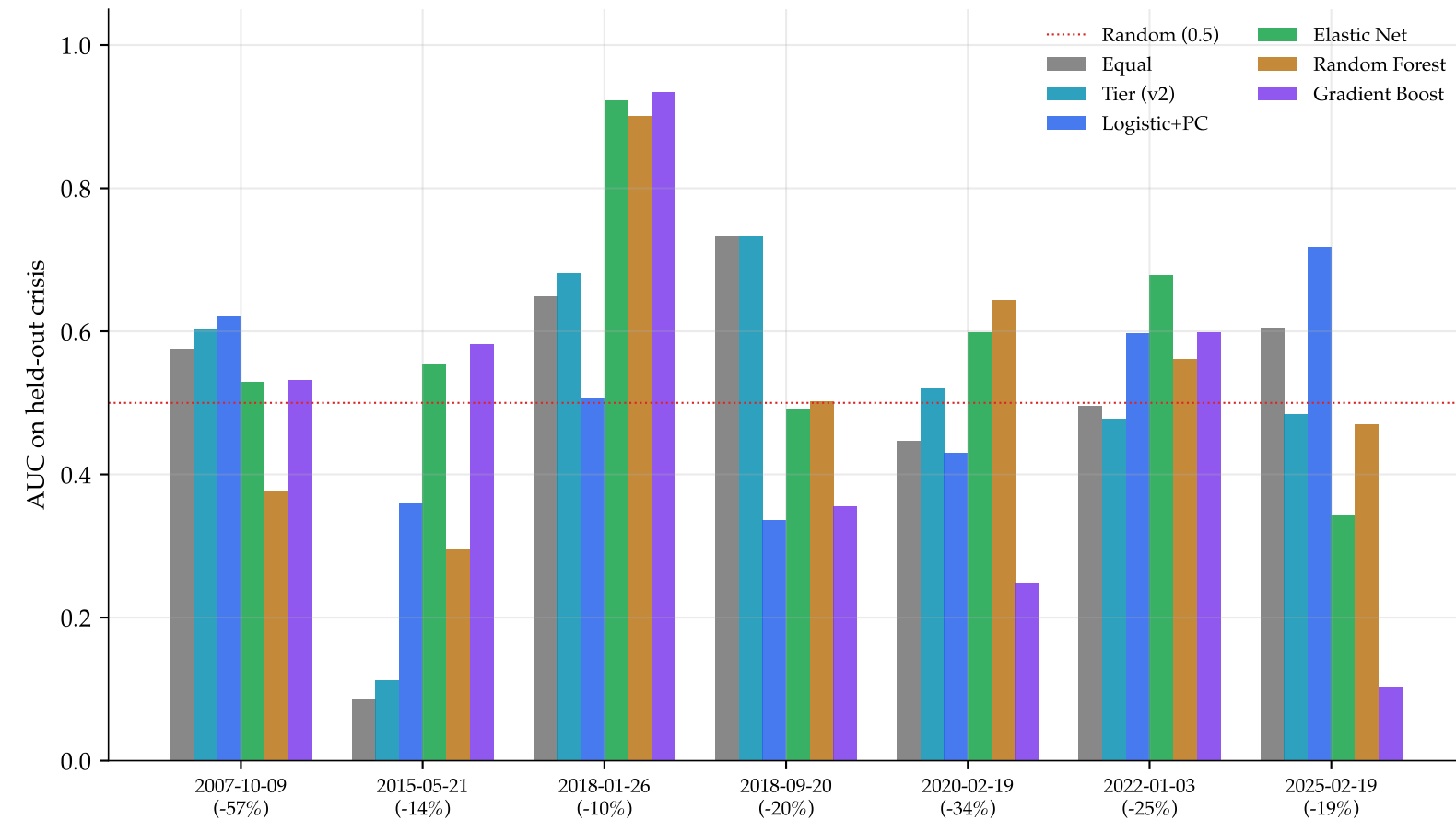
Per-crisis AUC (leave-one-crisis-out)
