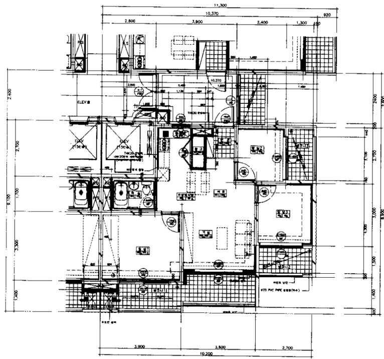
25층형 타워B형 단위평면도
