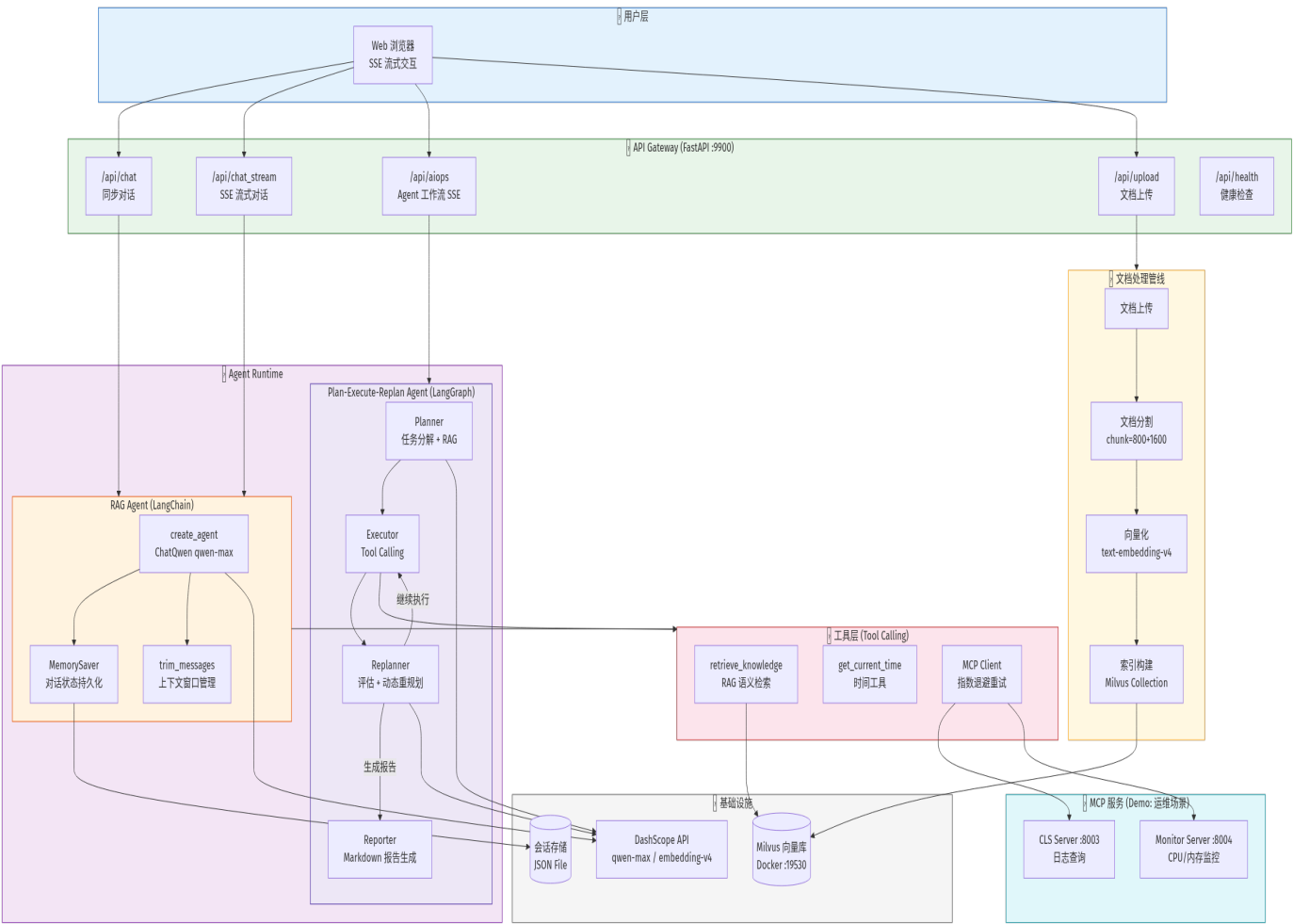
图 1: ReActLab 系统架构总览 — 从 Web 层到基础设施的完整数据流
