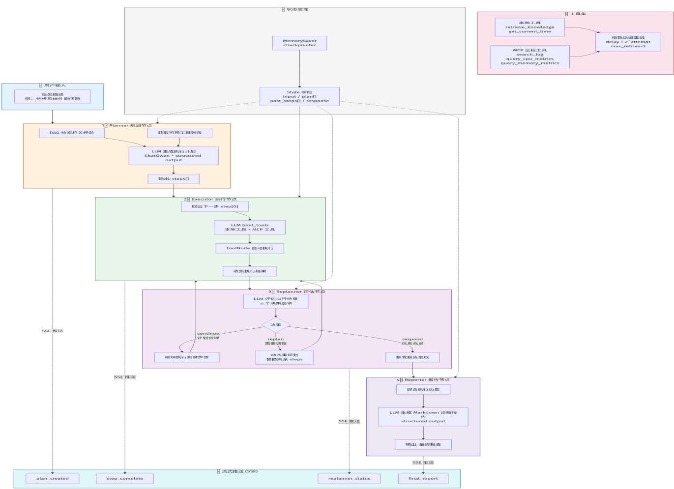
图 2: Agent Runtime workflow — Plan-Execute-Replan 循环 + 报告生成
