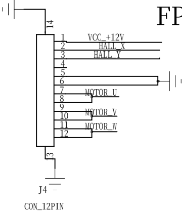
马达接口
