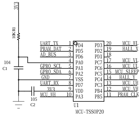
MCU
