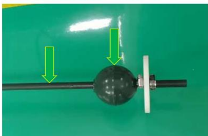
B. 定制护套管与浮球间隙的合理设计
