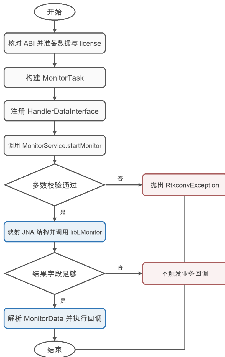
图 1 MonitorService 推荐接入流程
