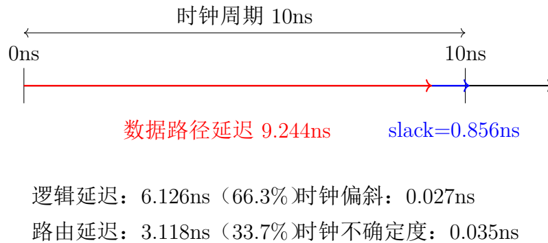
图 6: 最差路径建立时间分析示意图
