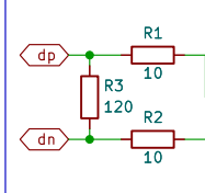
RS-485/RS-422 Terminations
