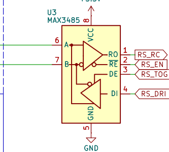
RS-485/RS-422 Transceiver
