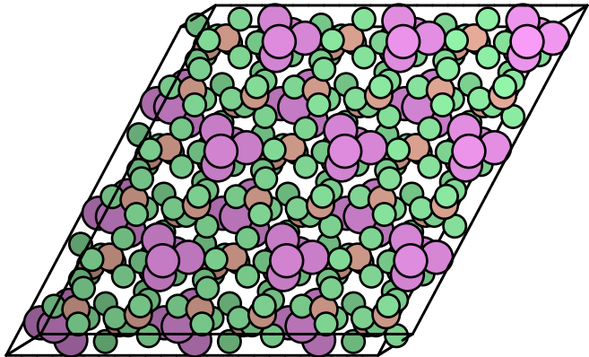
\text{Bi}_5\text{Ga}_3\text{Cl}_{12}
