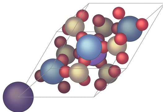
\text{Na}_2\text{O}_{24}\text{P}_6\text{Sn}_4
