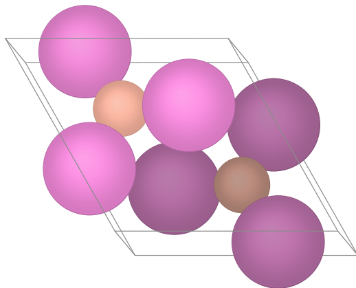
\text{B}_2\text{I}_6
