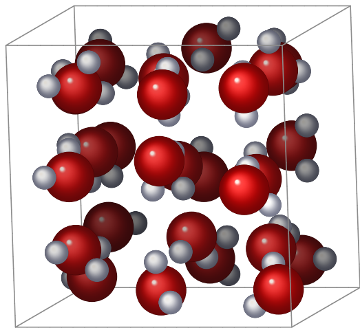
H54O27
