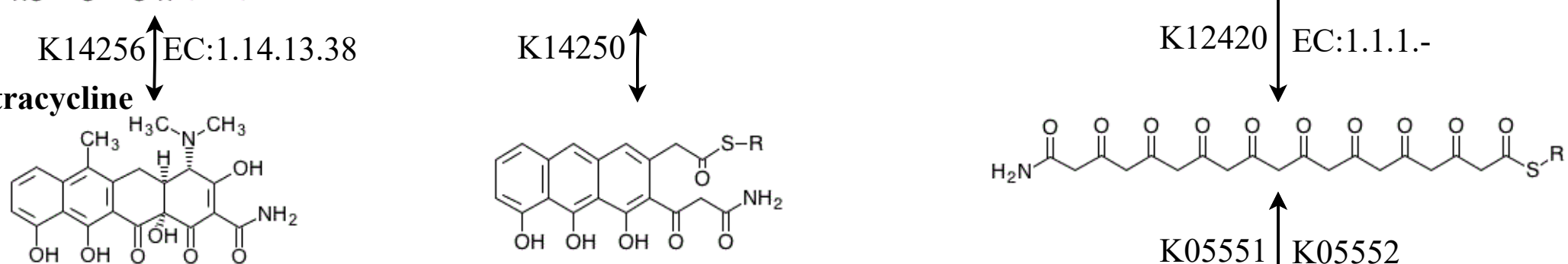
Malonamoyl-[acp]
