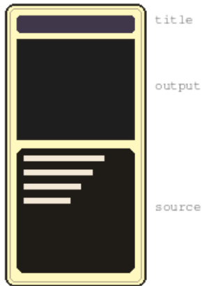
Figure 8: 三种布局策略。纵向：标题/图像/源代码从上到下堆叠，针对手机屏幕和纵向打印优化。横向：图像在左，标题和源代码在右，适合横向卡片和并排浏览。明信片：正面是渲染输出，背面是源代码和元数据——一张可邮寄的卡片，翻转后才能看到程序。
