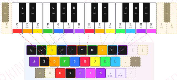
Figure 1: notepat.com 的键位映射。QWERTY 字母 C 弹奏 C , D 弹奏 D , ..... , B 弹奏 B ; 上方八度继续按字母排列 ( H I J K L M N ) ; 升号尽可能依钢琴黑键的类比落在其本位音上方。双手分工 : 低八度归左手 (蓝色区域) , 高八度归右手 (粉色区域) ; 变暗的按键扩展音域。各实现 : notepat.com (网页) 、 AC Native OS、MenuBand ( macOS 菜单栏 ) 、 Ableton ( Max for Live ) 插件、babypat。
