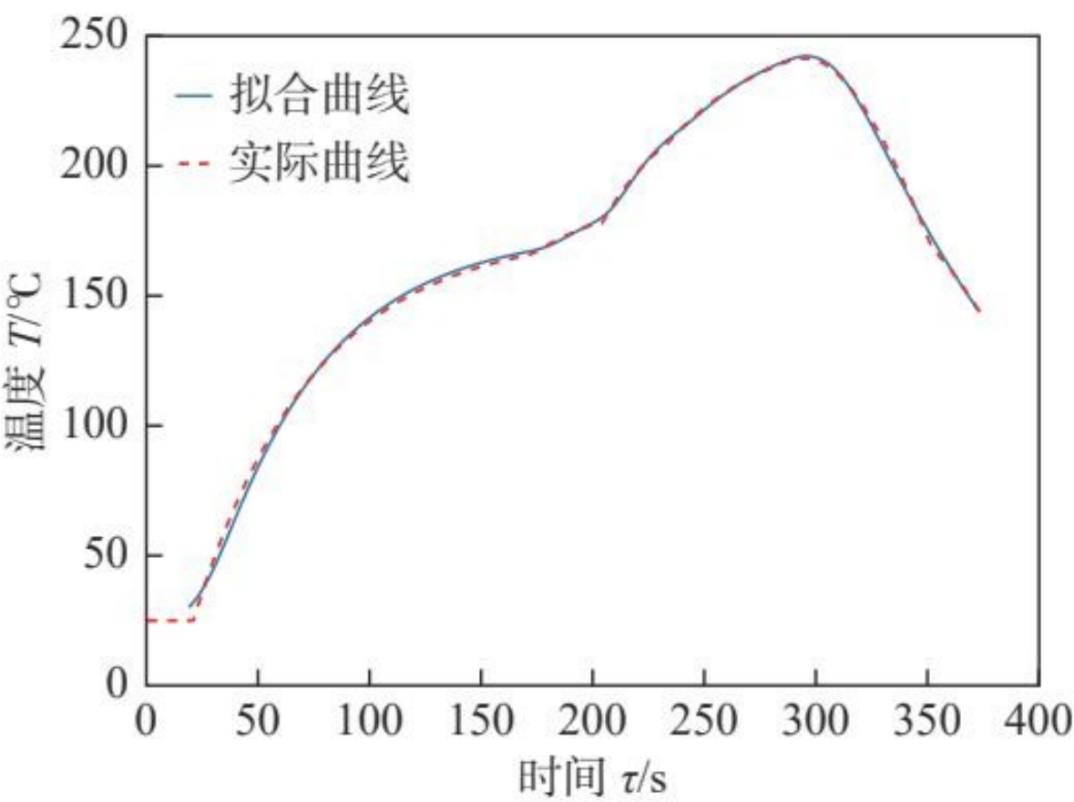
模拟炉温曲线与实测温度曲线对比
