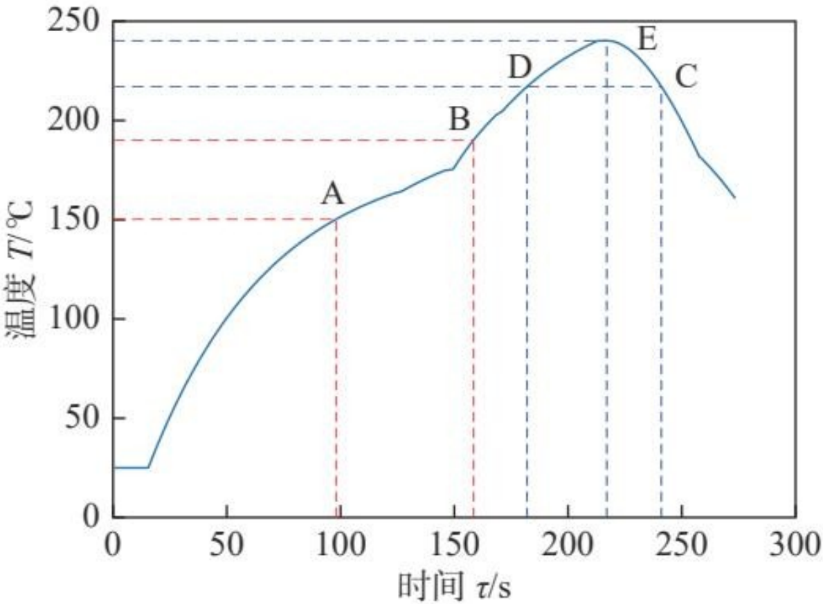
优化后的炉温曲线（A-E 特殊点标注）
