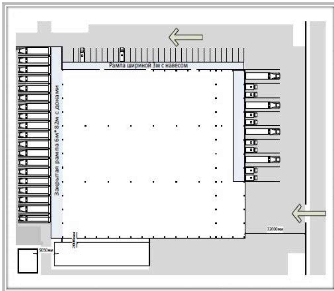
План 1 этажа
