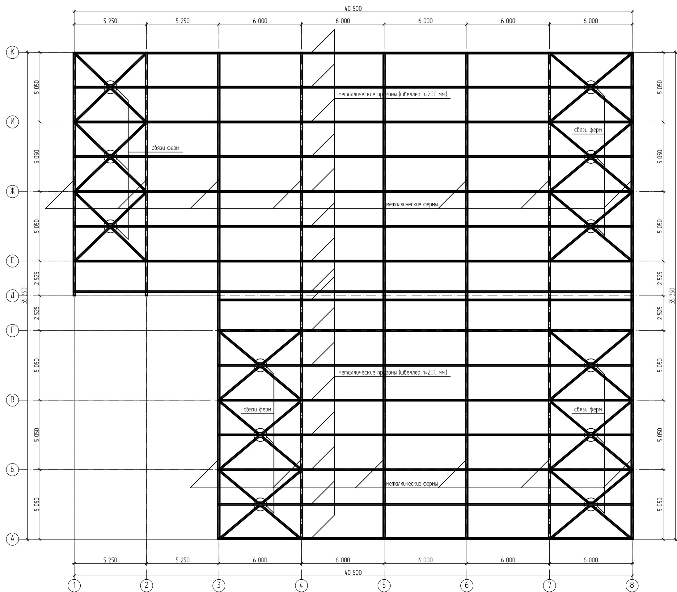
Схема расположения металлических ферм, прогонов и связей. М 1:200.
