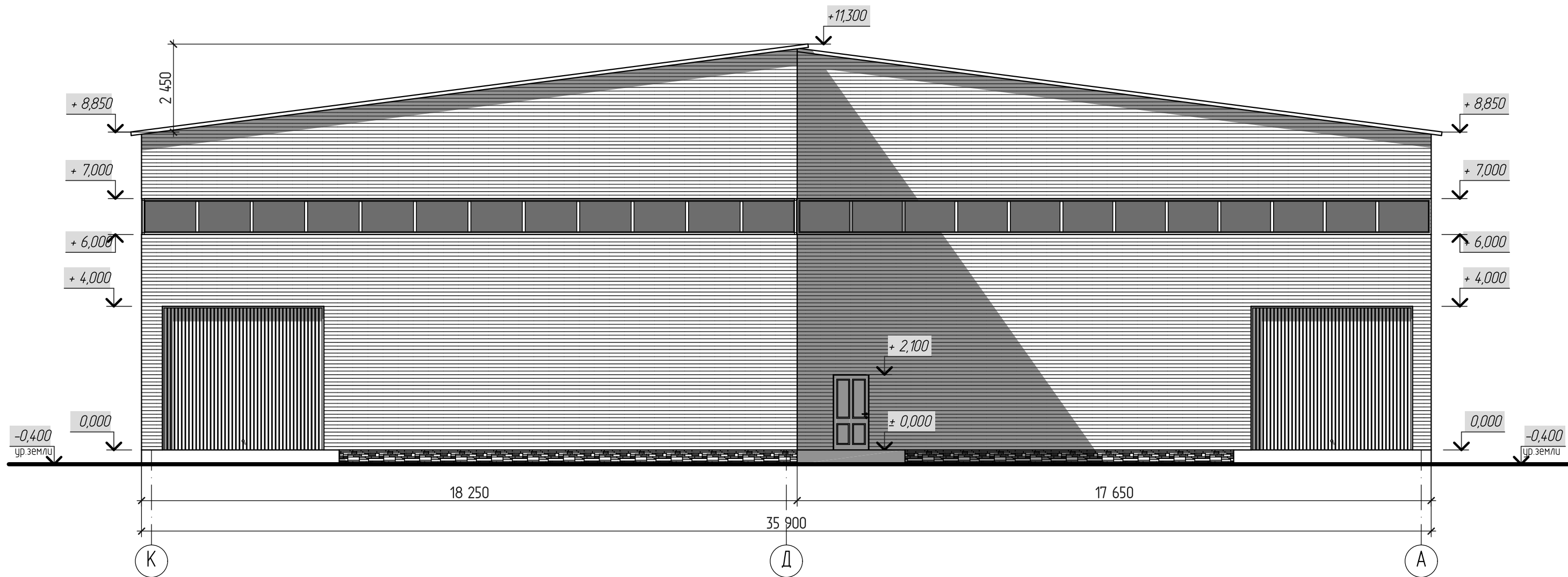
Фасад "К-А". М 1:100.
