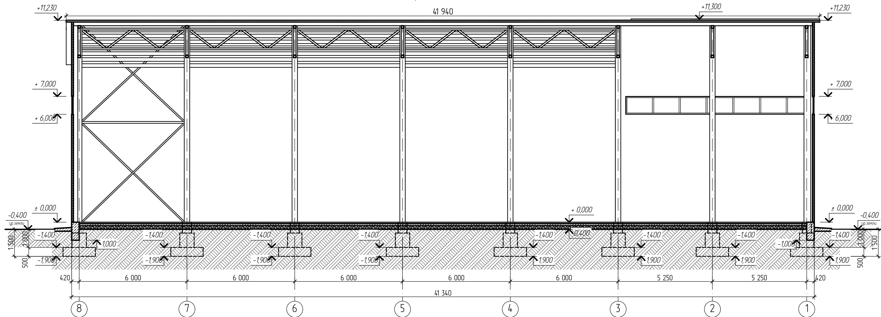
Разрез 2-2. М 1:150.
