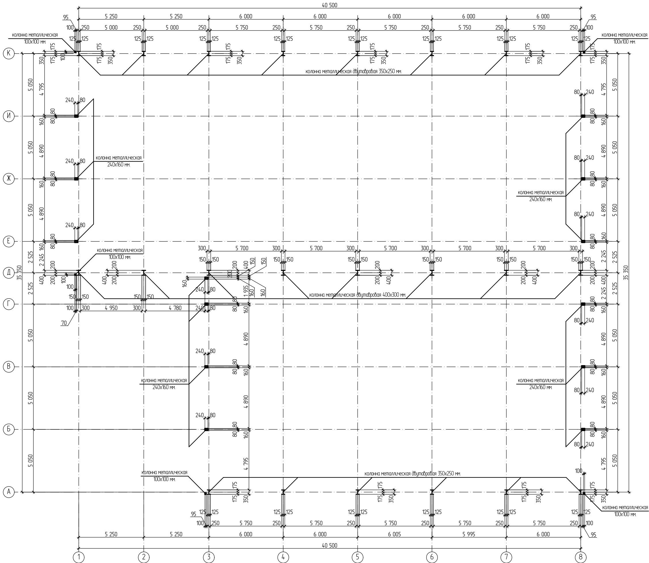
Схема расположения металлических колонн на отм. +0.000. М 1:200.
