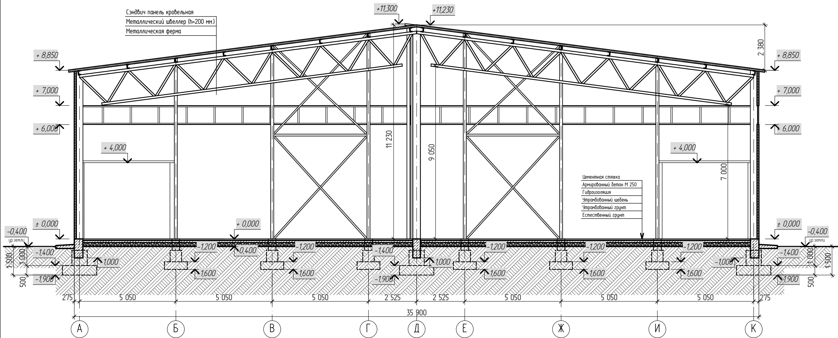
Разрез 1-1. М 1:100.
