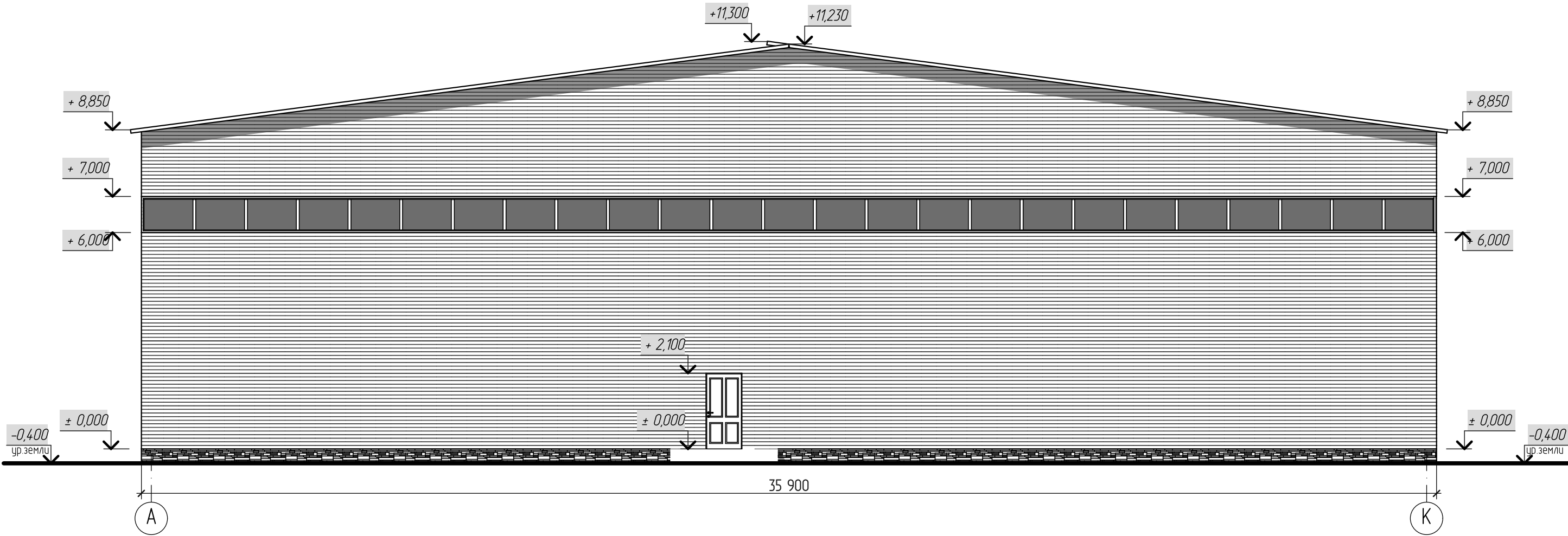
Фасад "А-К". М 1:100.
