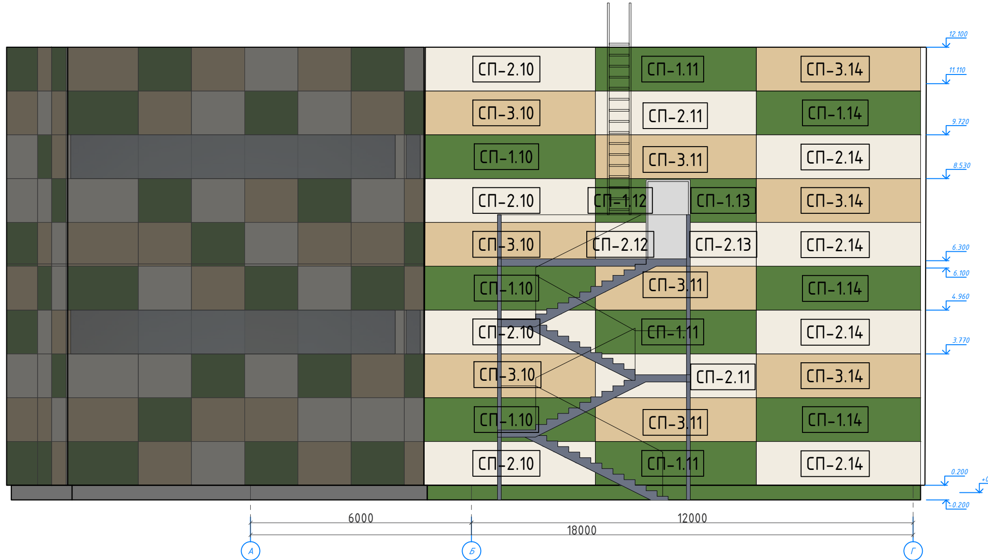
Фасад А-Г, М 1:10
