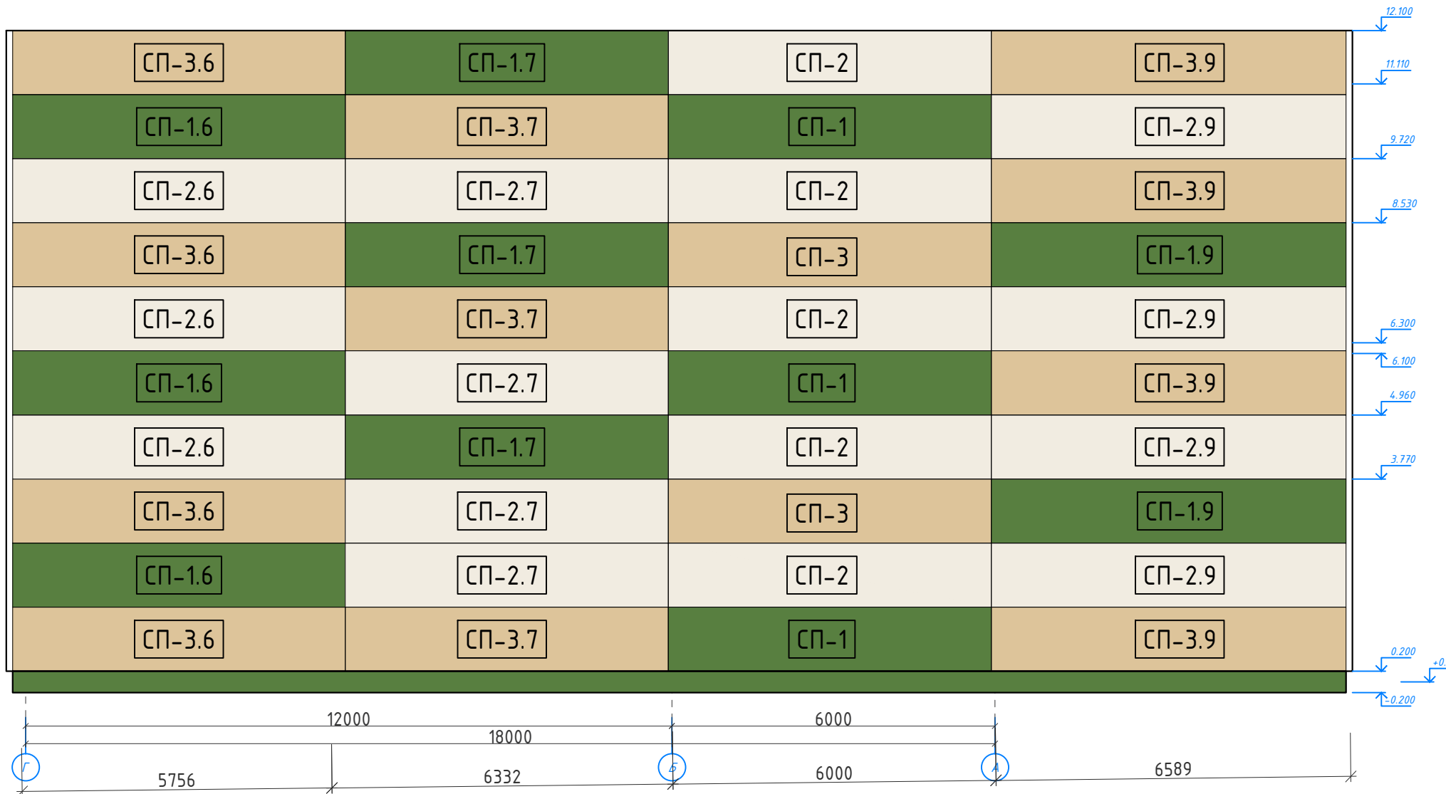
Фасад Г-А, М 1:10
