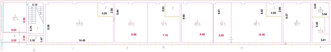
Масштаб 1:200
