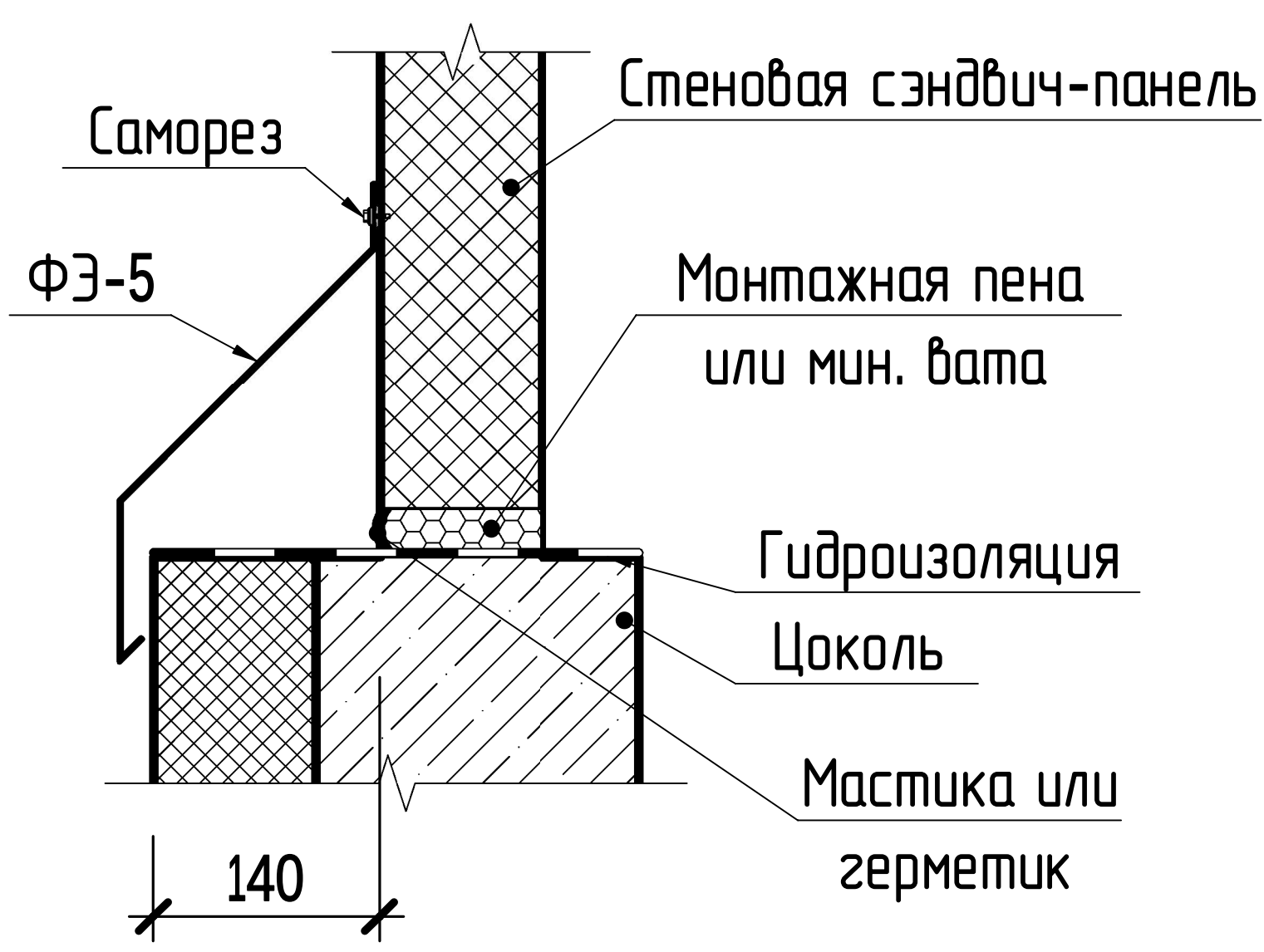
Примыкание сэндвич-панели к цоколю
