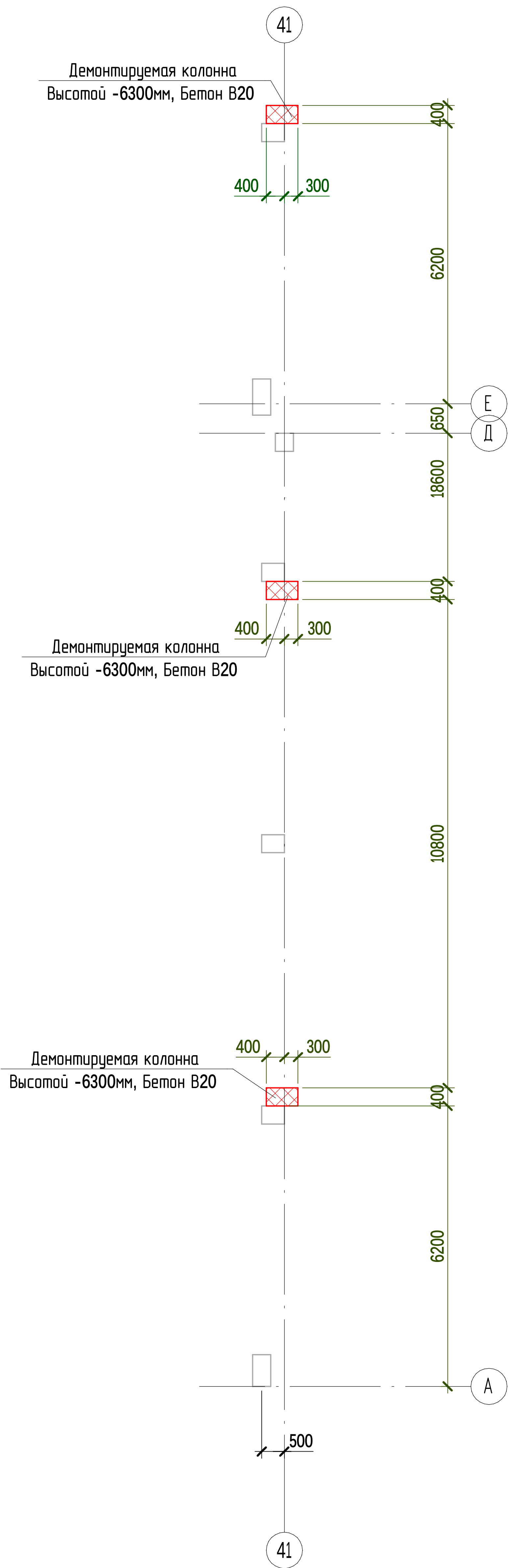
Схема расположения колонн по оси 41 (демонтаж) ( 1 : 100)
