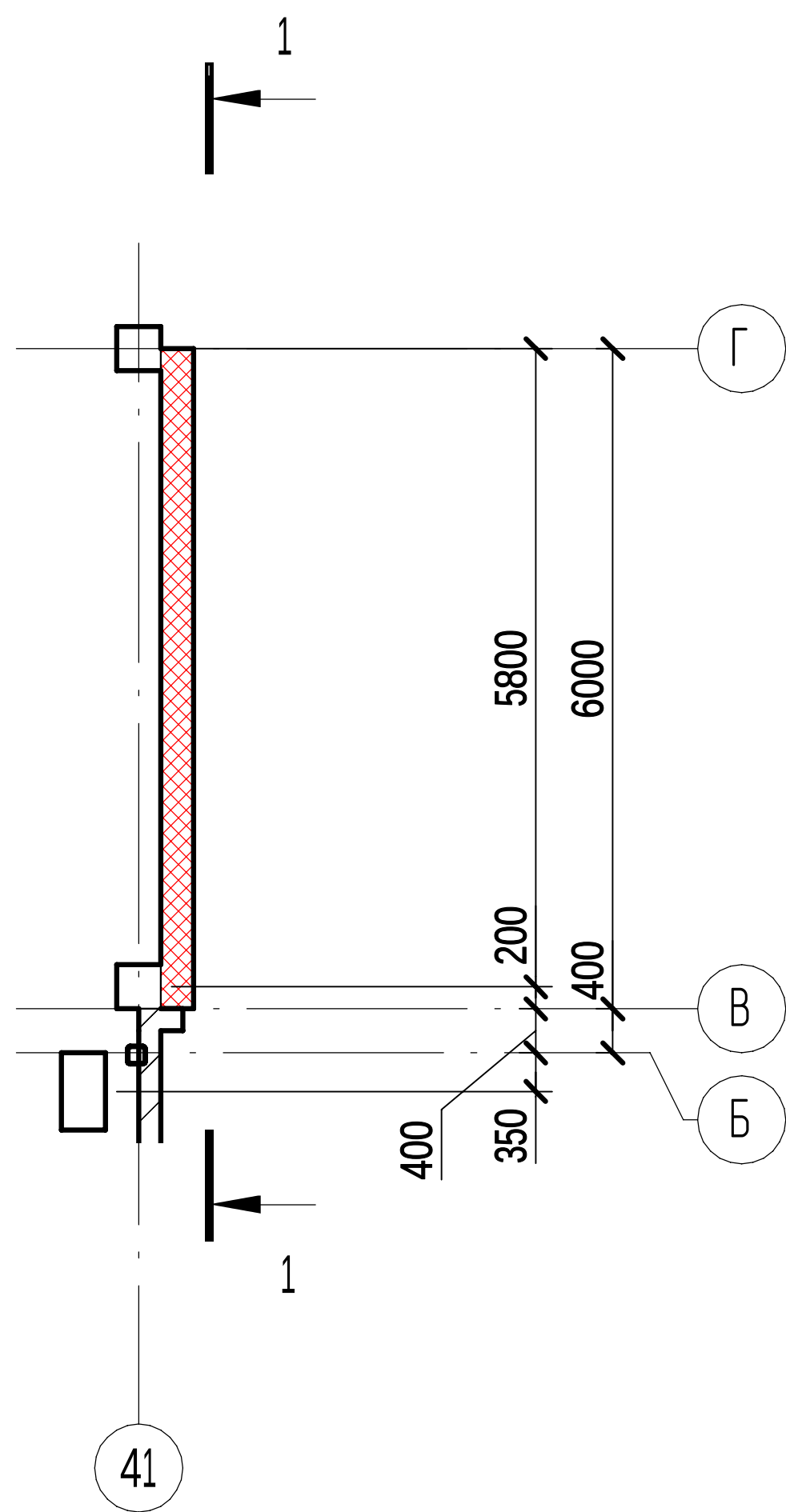
Схема расположения стен по оси 41 (демонтаж) ( 1 : 100)
