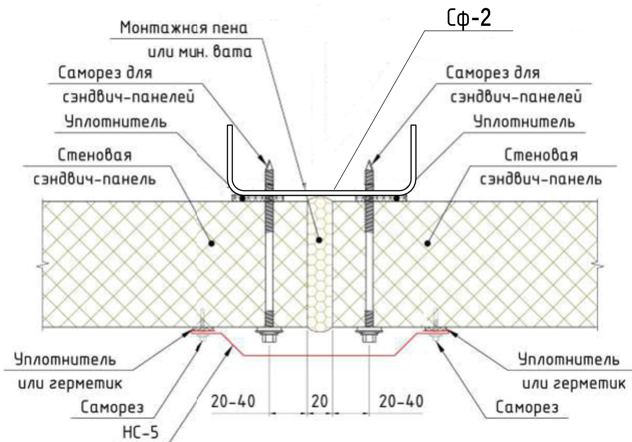
Стык сэндвич-панелей по колонне
