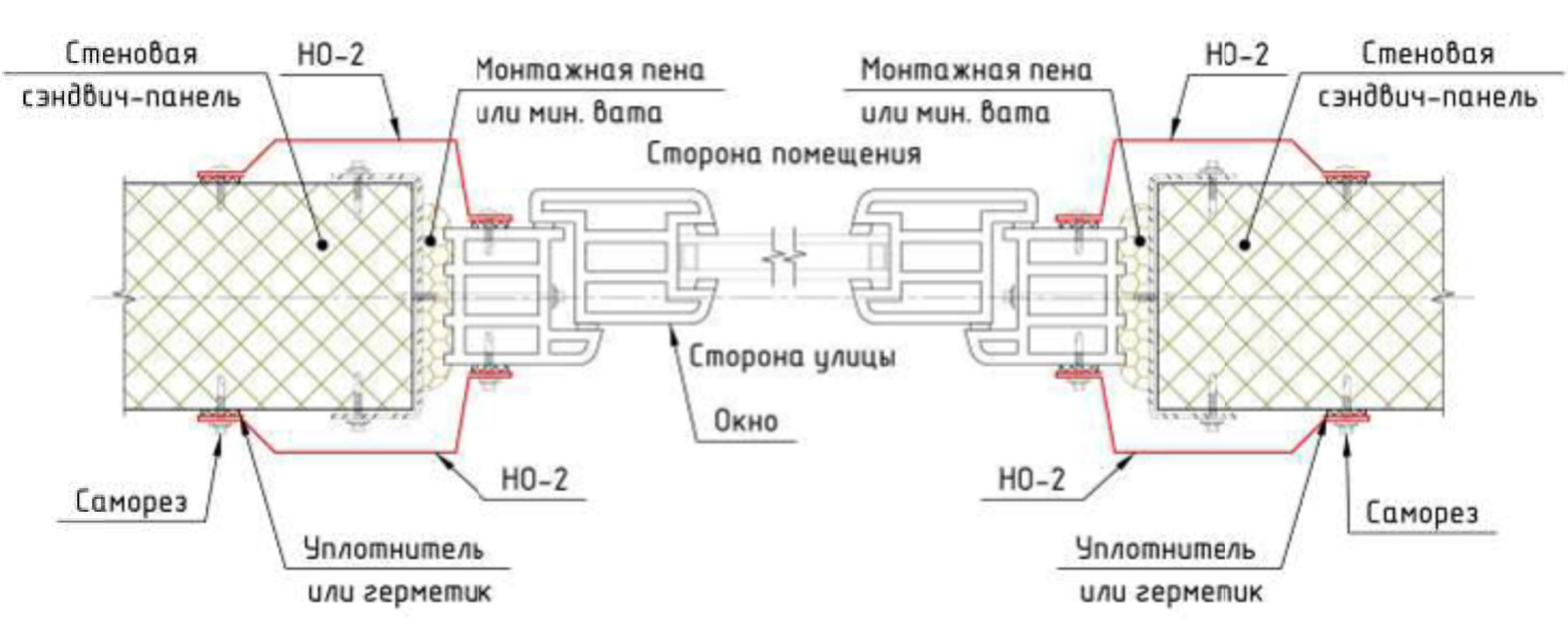
Обрамление оконных блоков из ПВХ
