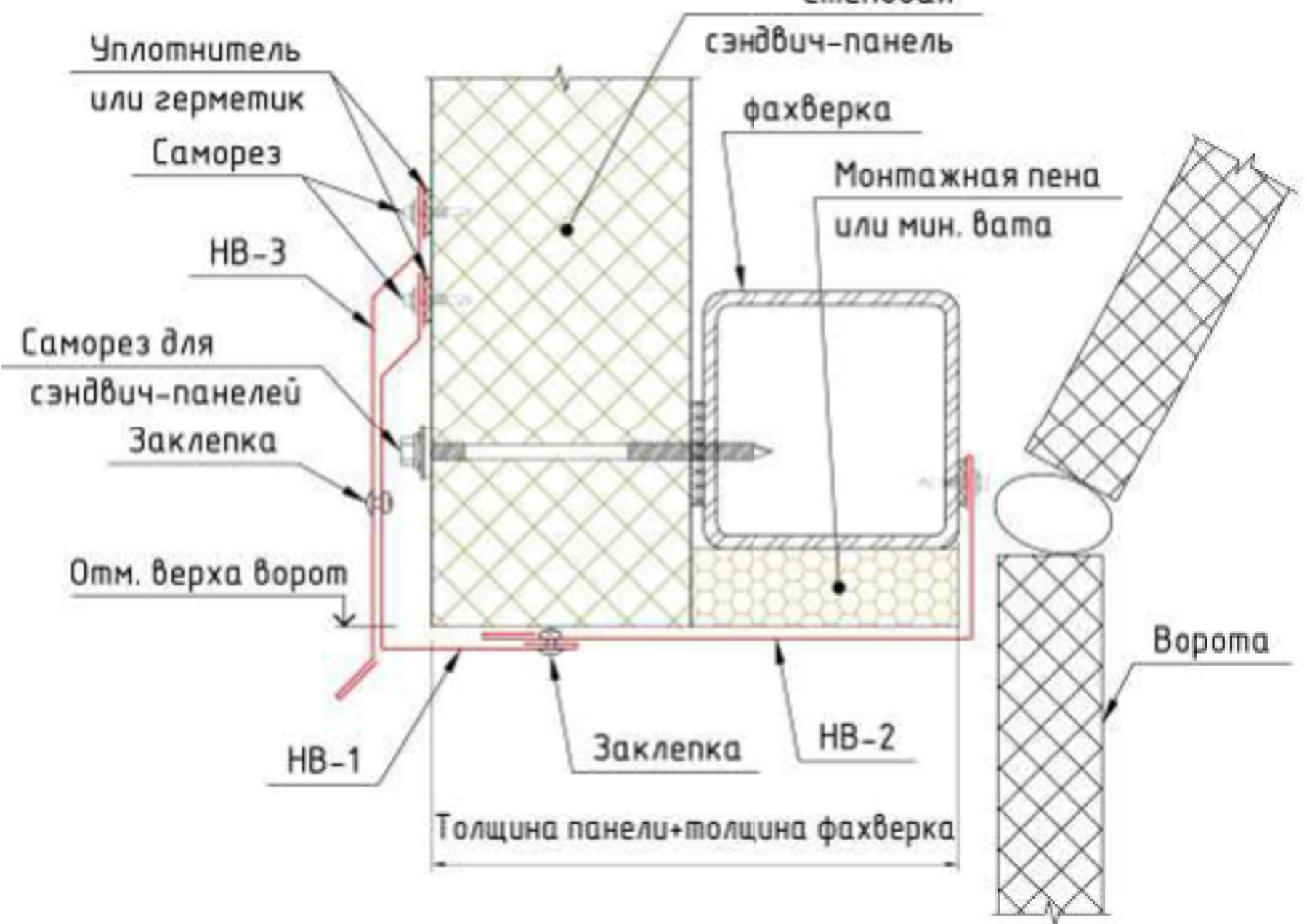
Обрамление секционных (подъемных) ворот
