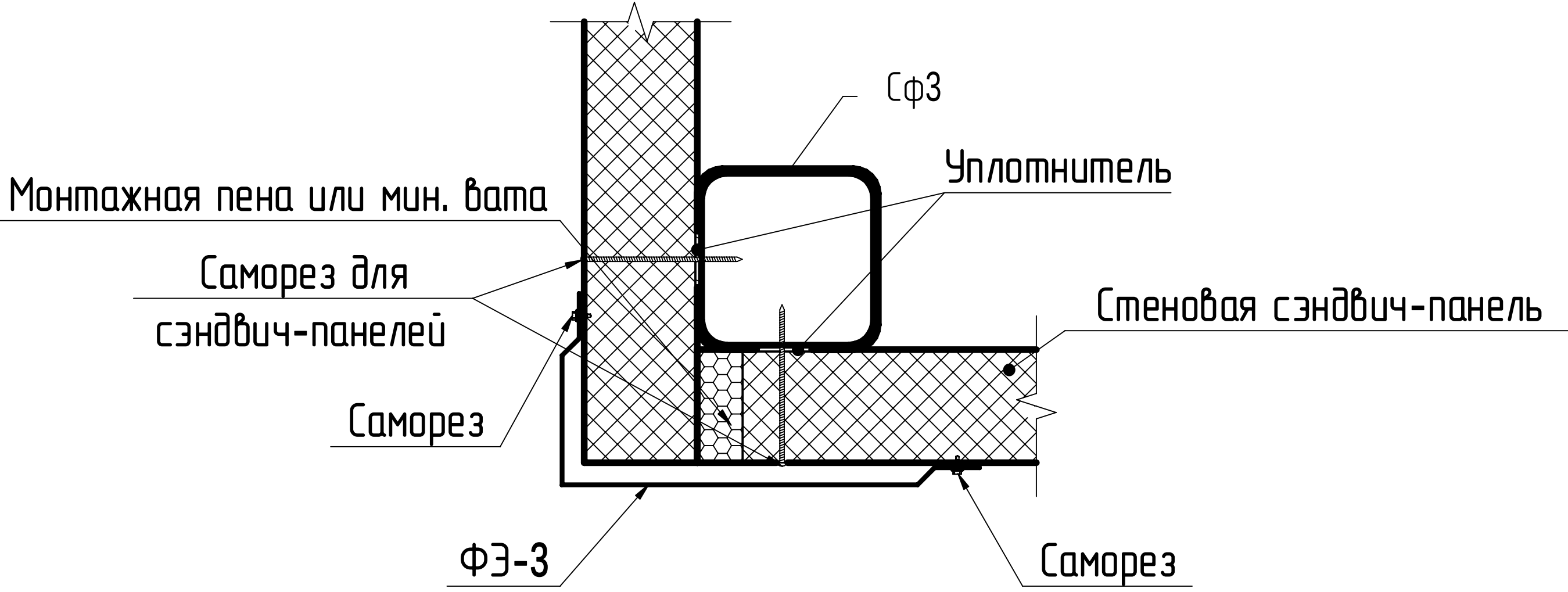
Стык сэндвич-панелей по внешнему углу
