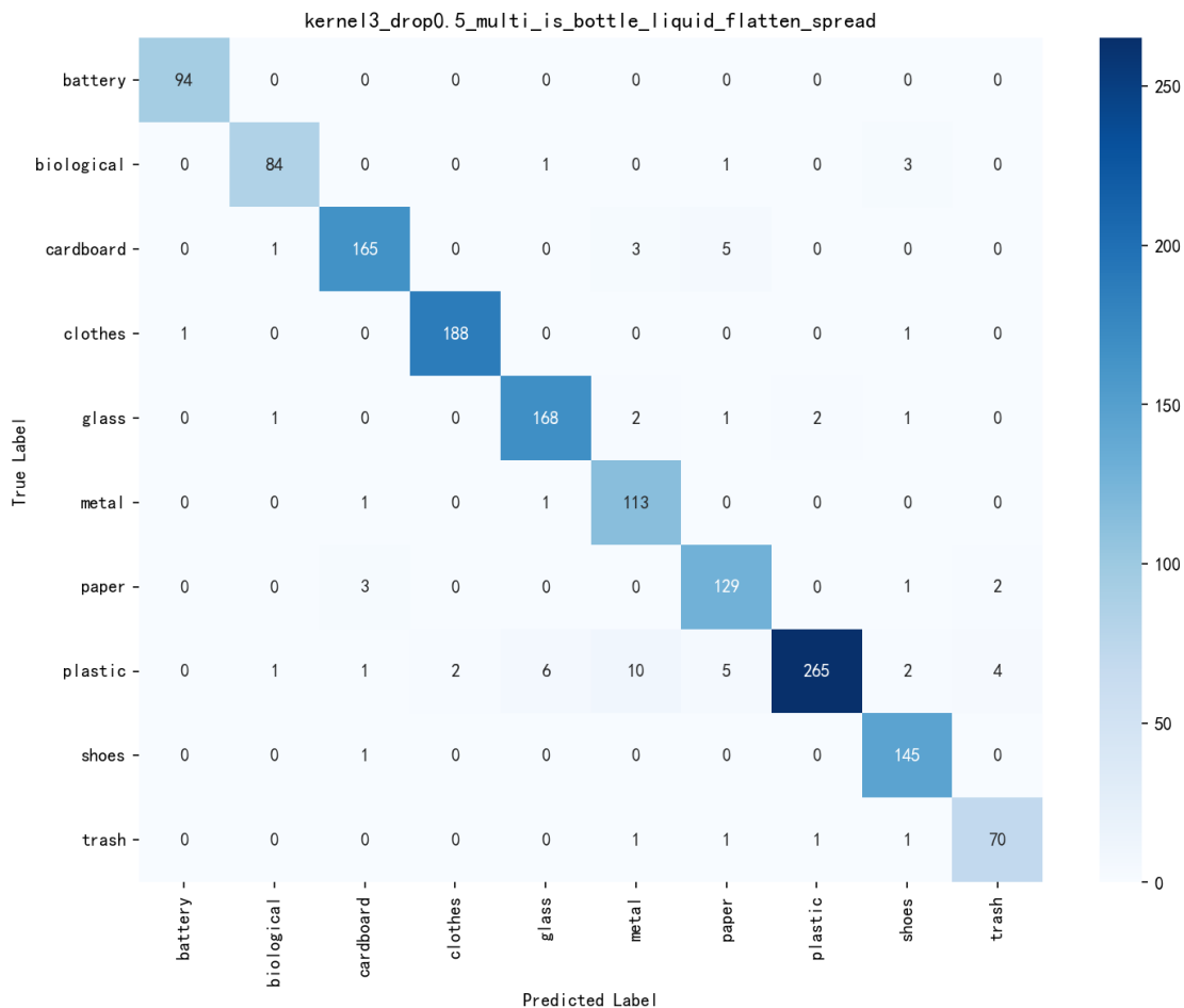
图 5: 测试集混淆矩阵
