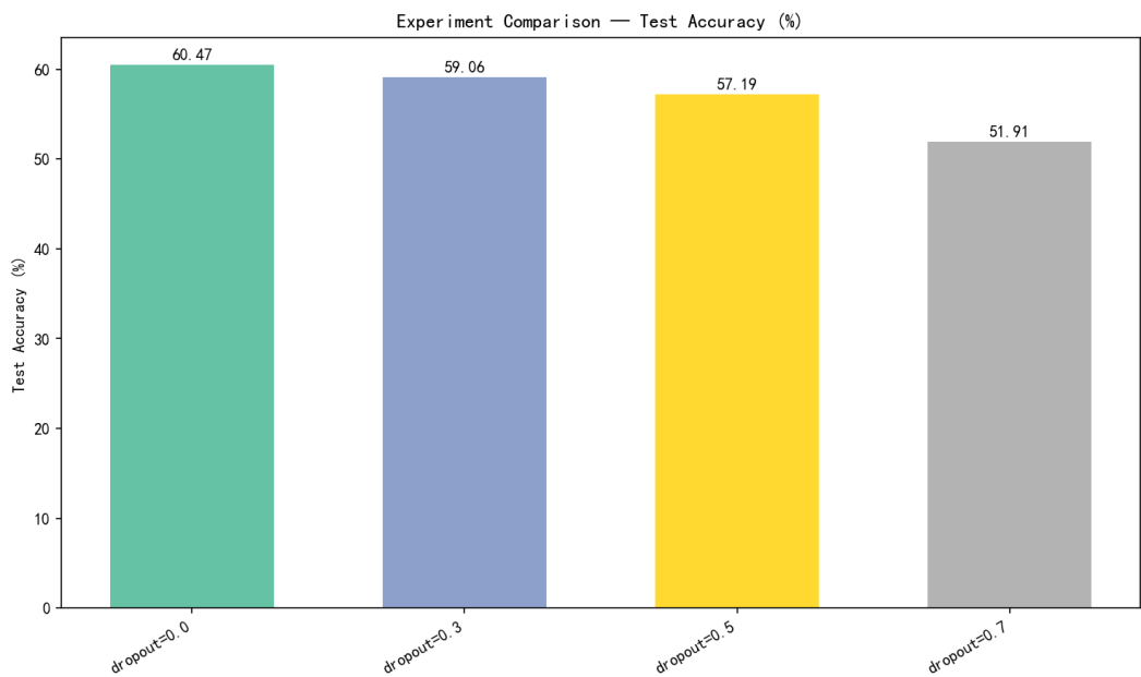
图 7: Dropout 比例对比实验结果
