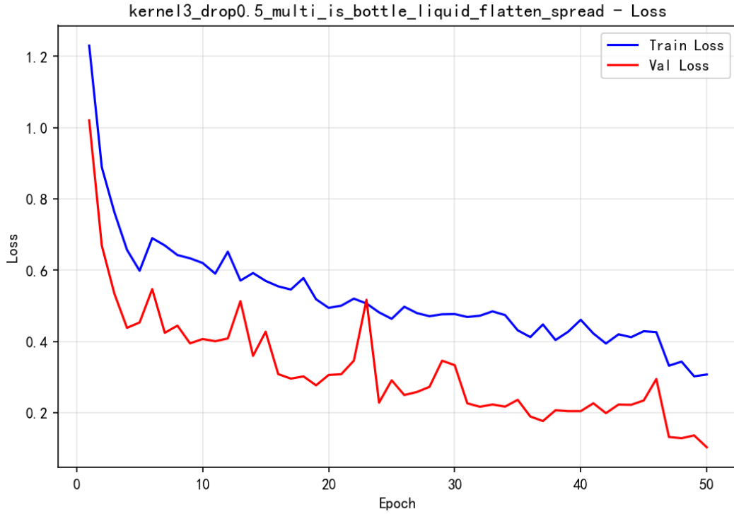
图 3: 训练 Loss 曲线（蓝 = 训练集，红 = 验证集）
