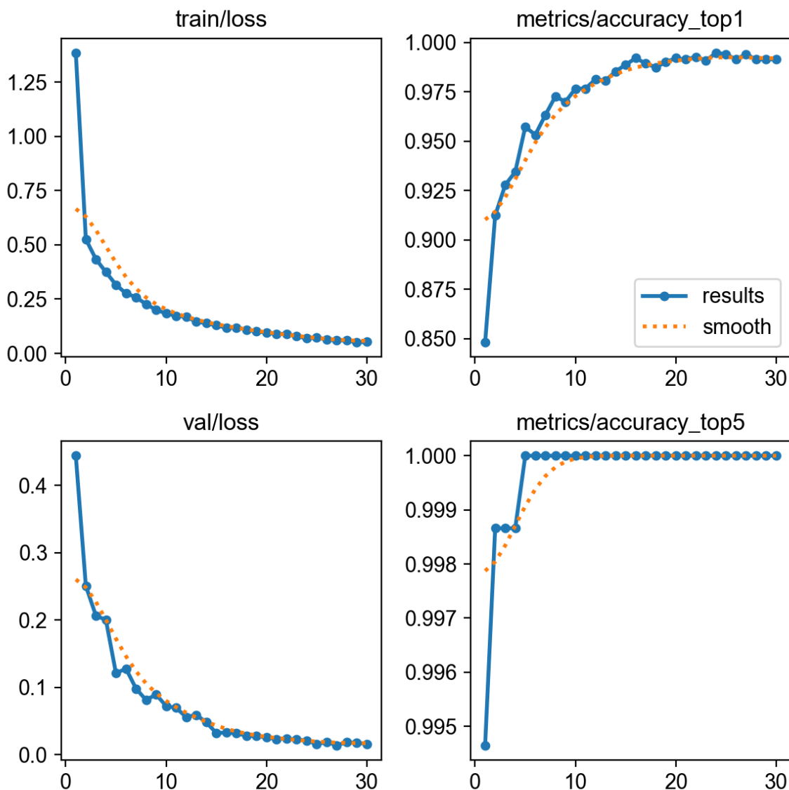
图 9: YOLOv8n-cls 训练曲线 (30 epochs)
