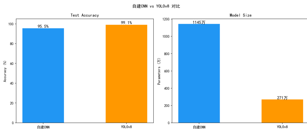
图 8: 自建 CNN vs YOLOv8 准确率与参数量对比
