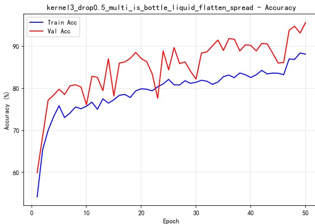
图 4: 训练 Accuracy 曲线 (蓝 = 训练集, 红 = 验证集)
