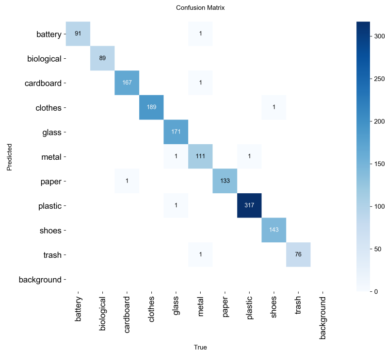
图 10: YOLOv8n-cls 测试集混淆矩阵
