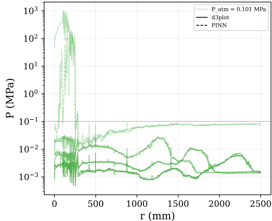
R_0=100\text{mm} — P(r) profiles
