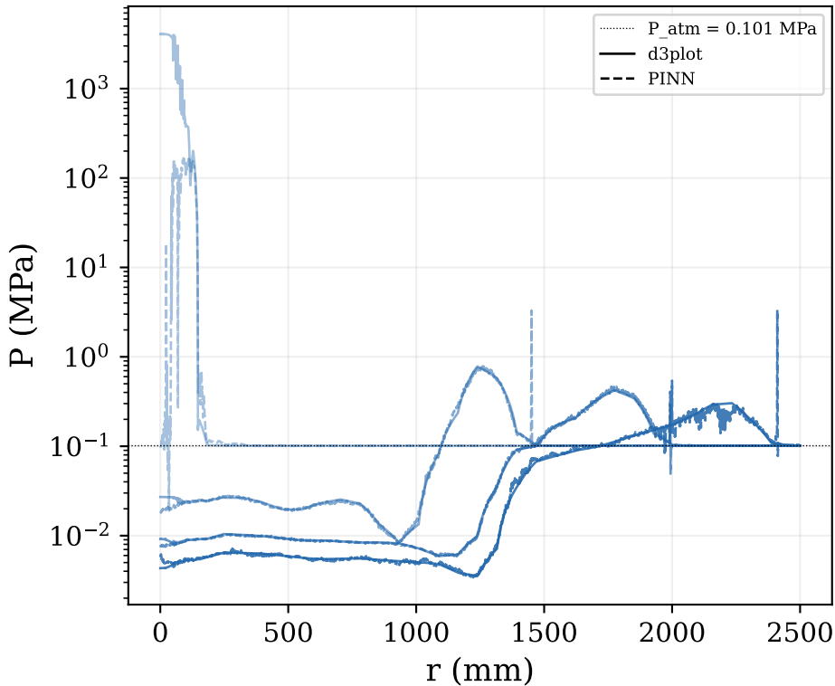
R_0=50\text{mm} — P(r) profiles
