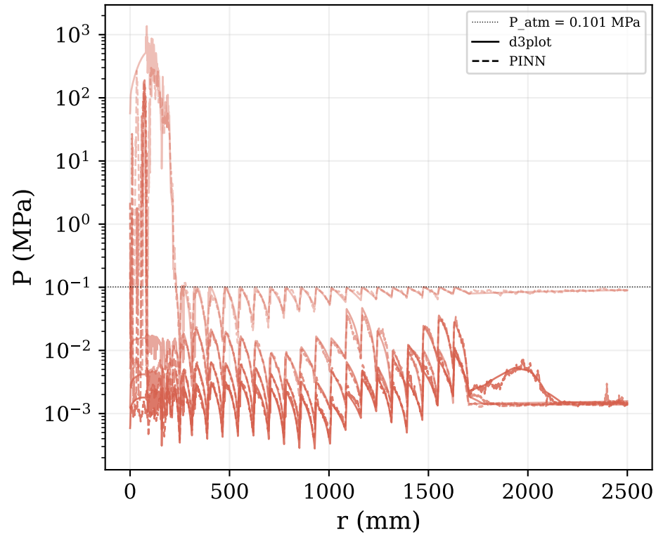
R_0=80\text{mm} — P(r) profiles
