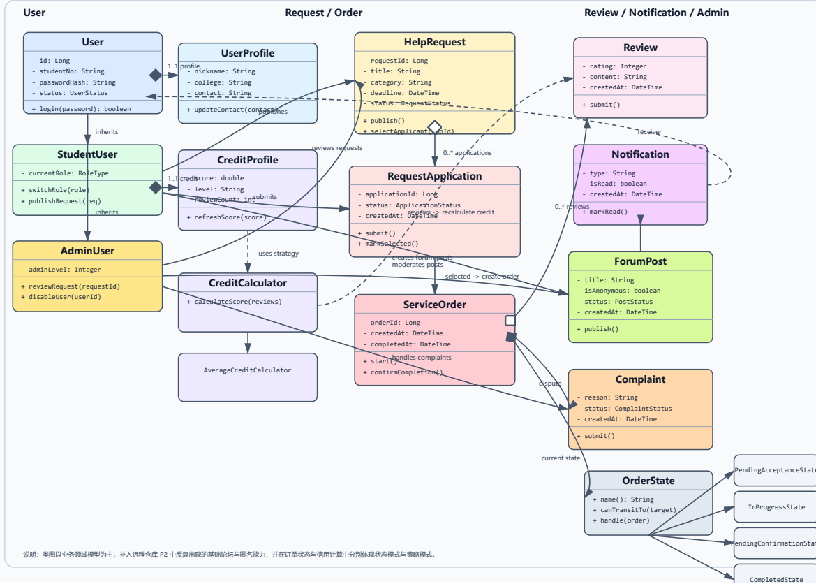
CampusHub 核心类图
