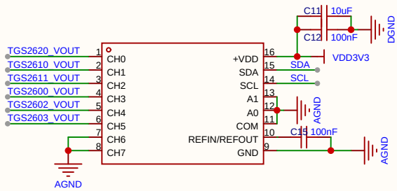
ADC
