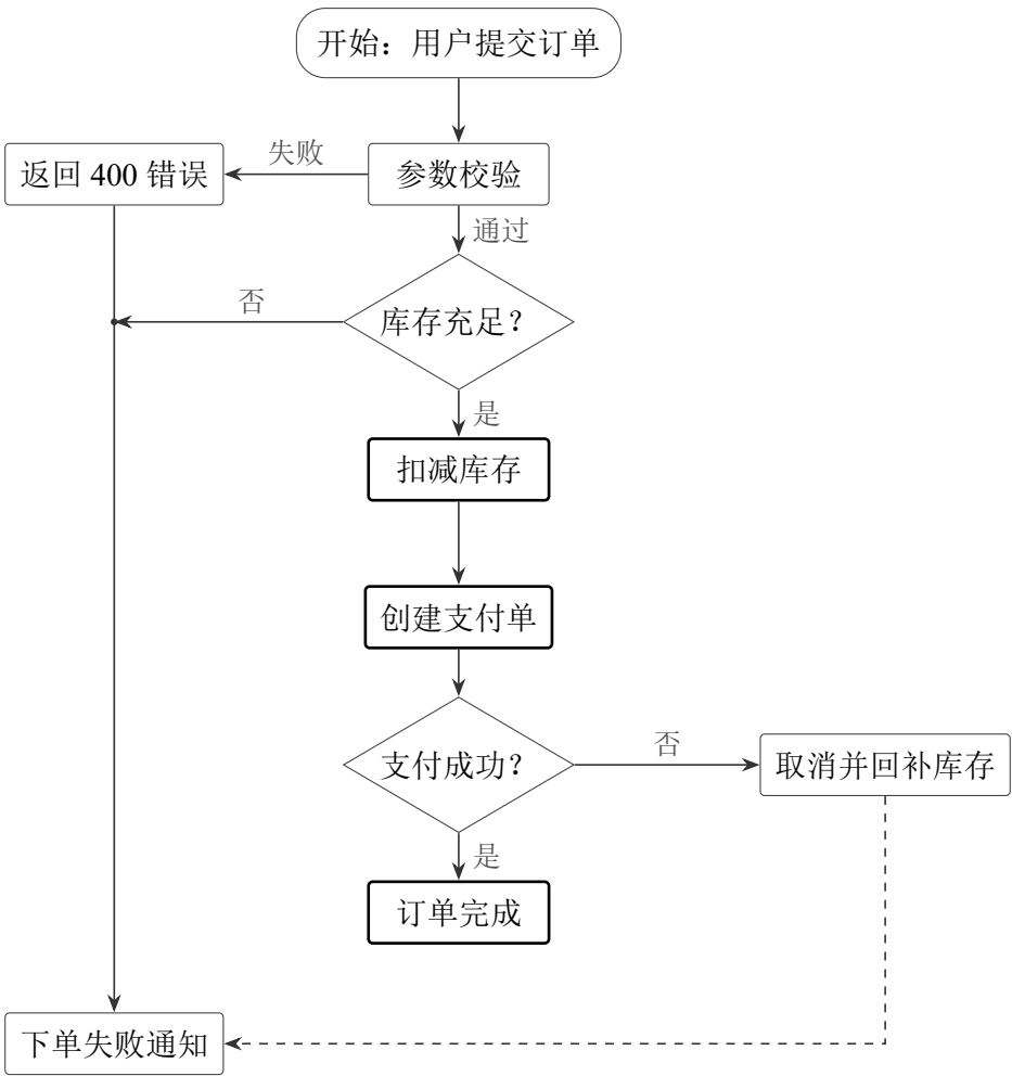
图 3.1 订单处理流程
