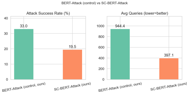
图 3 自实现 BERT-Attack 与 SC-BERT-Attack 对比
