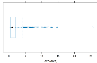
(d) Boxplot
