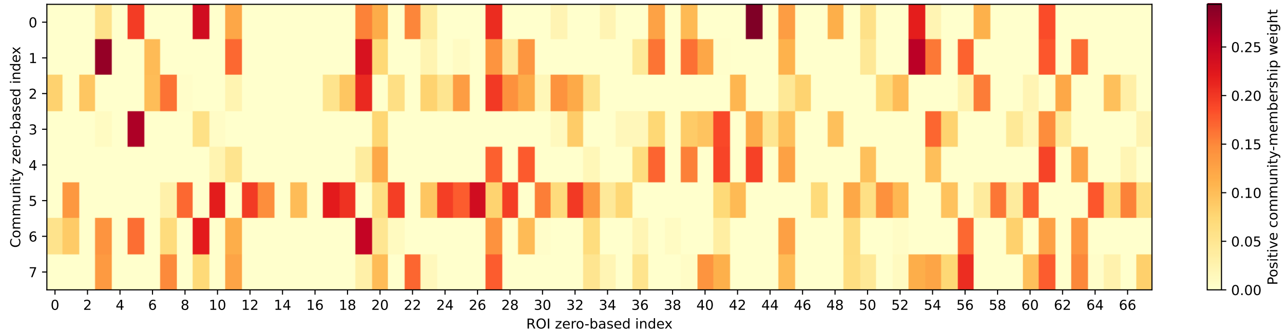
图 3.8 第一层 Ra-GConv alpha+ 矩阵 (fold_3)
