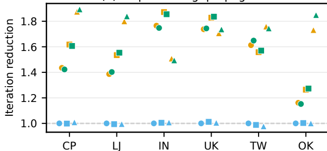
(d) Preprocessing: propagation
