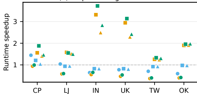
(d) Preprocessing: propagation
