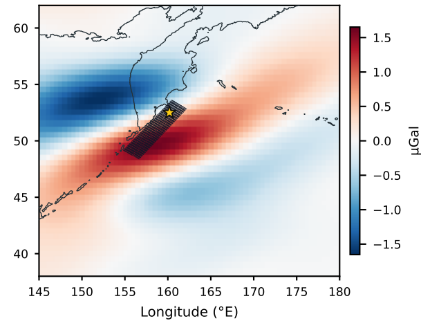
(d) GNSS GRACE-FO-resolution radial gravity
