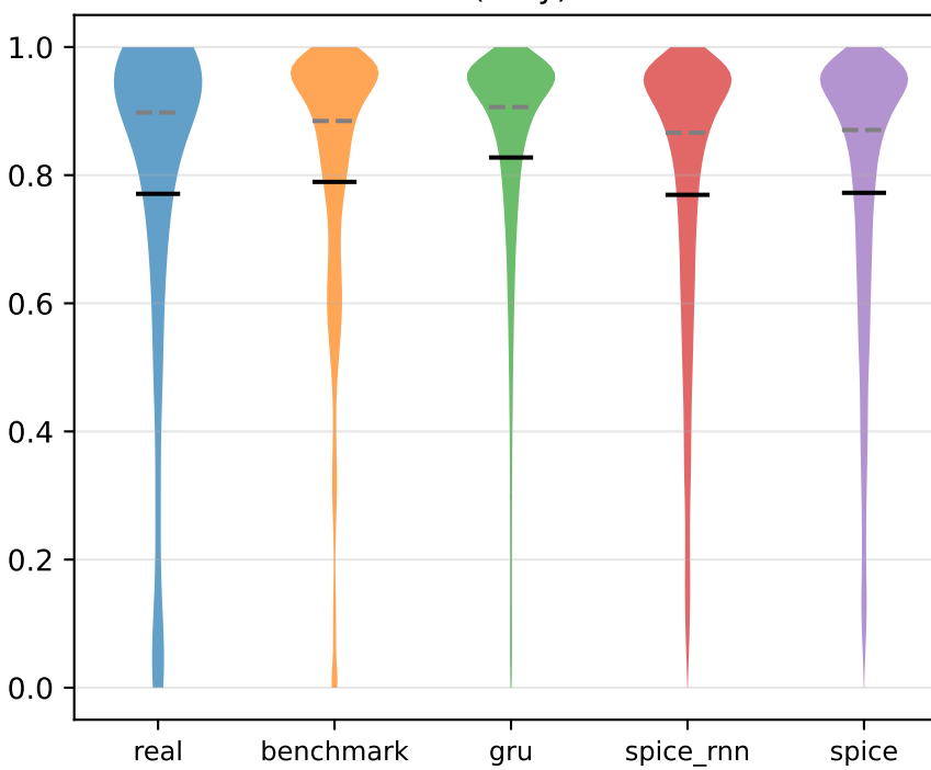
P(Stay)
