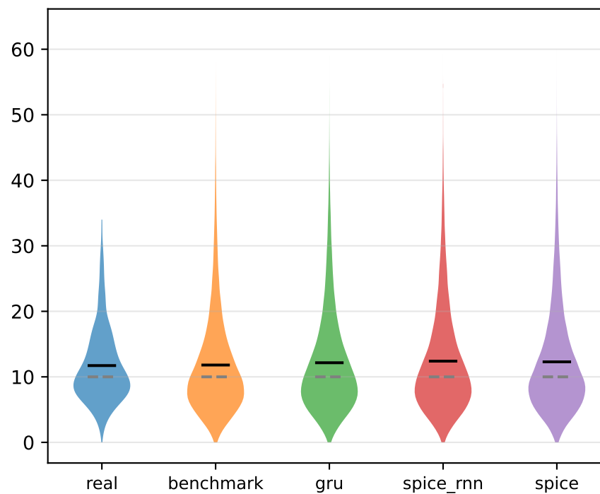
P(Stay)
