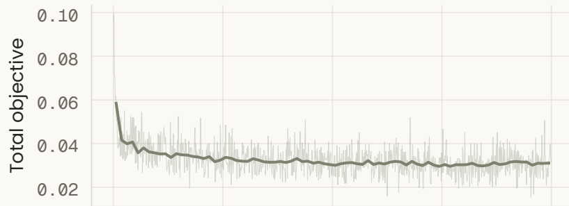
DnCNN
