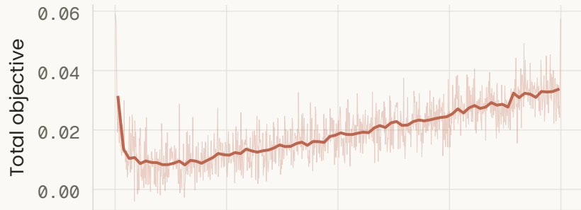
FCSG-Net
