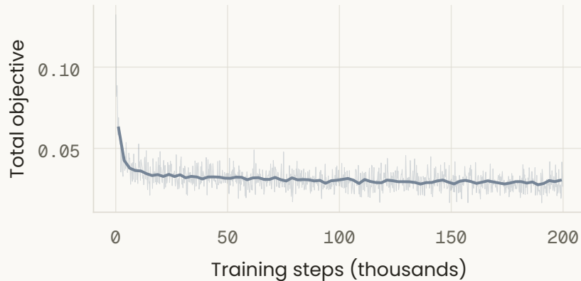
FFDNet oracle
