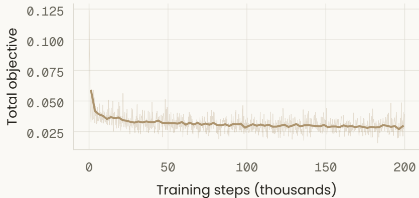
FFDNet blind
